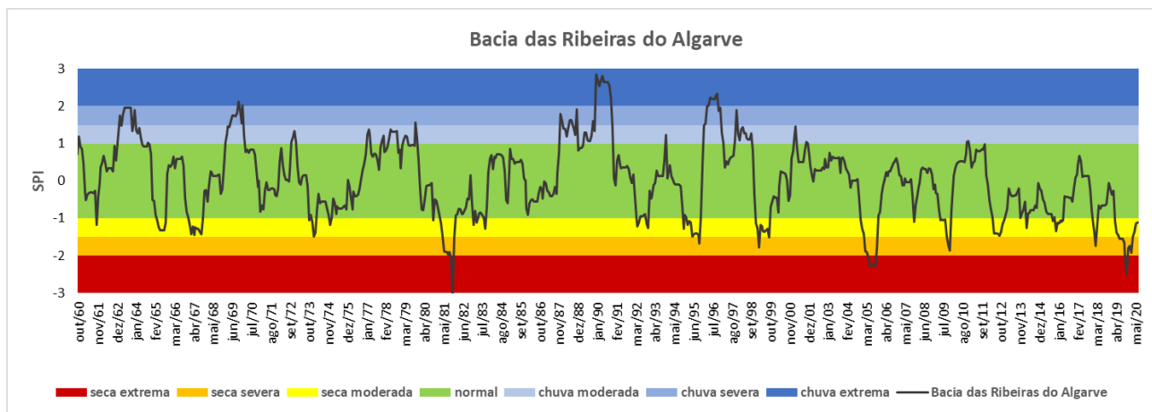
Figura 4.3 – Índice SPI-12 para a Região Hidrográfica do Algarve
