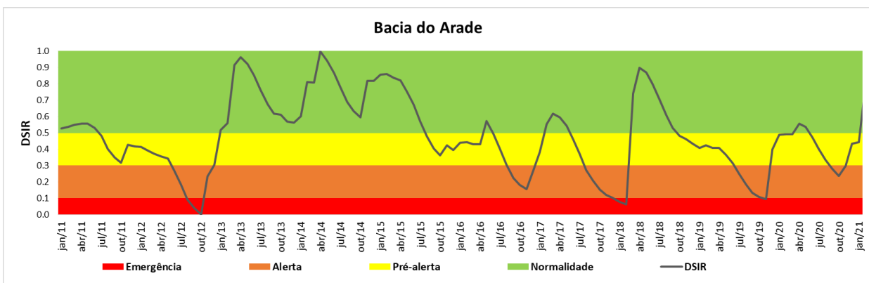
Figura 4.5 – Aplicação do índice Drought State Index for Reservoirs na Região Hidrográfica das Ribeiras do Algarve, Arade
