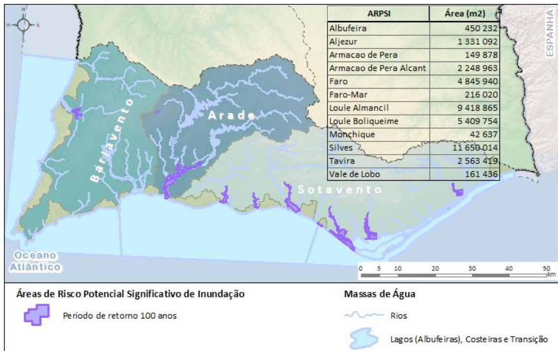
Figura 4.7 – Localização das ARPSI para a RH – 2.º ciclo
