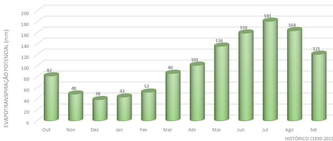
Figura 1.7 – Evapotranspiração média mensal na RH
