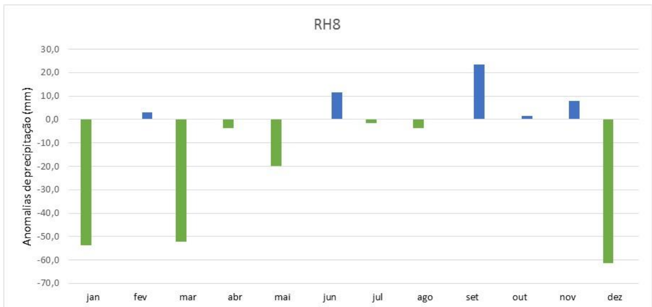
Figura 3.14 – Desvio da precipitação mensal no ano hidrológico 2020/21 para a RH
