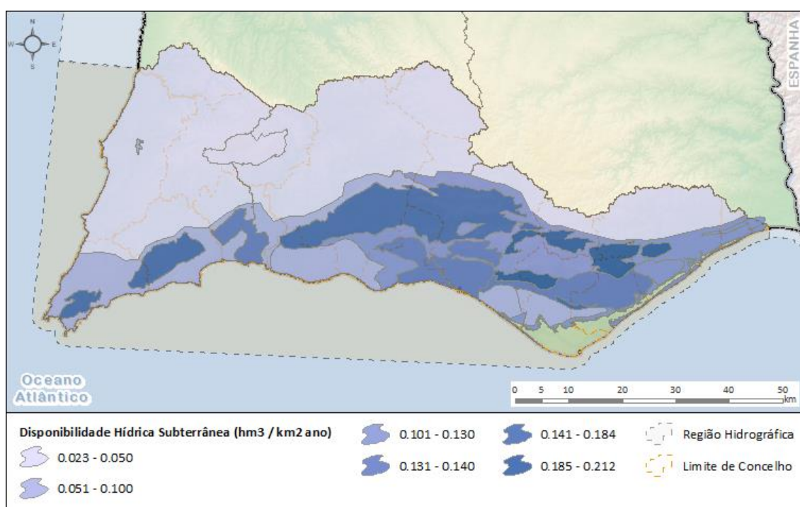
Figura 1.16 – Disponibilidade hídrica subterrânea por unidade de área na RH
