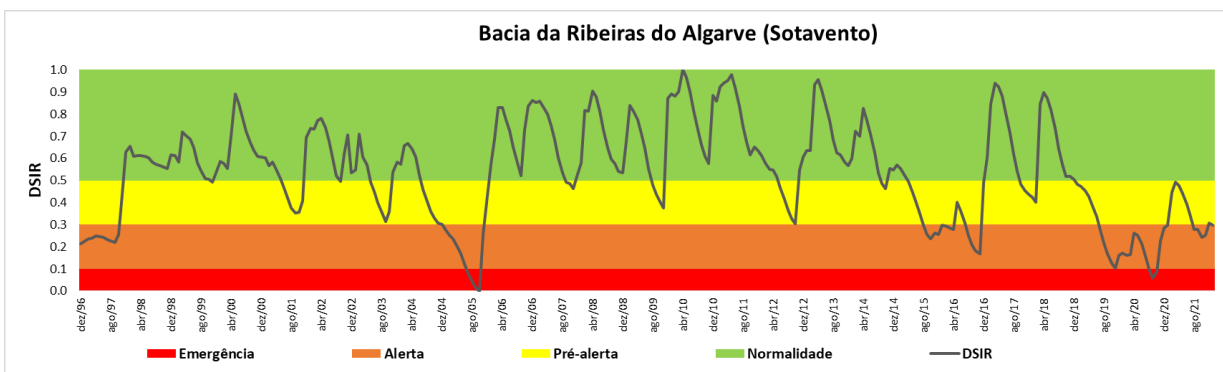
Figura 4.6 – Aplicação do índice Drought State Index for Reservoirs na Região Hidrográfica das Ribeiras do Algarve, Sotavento
