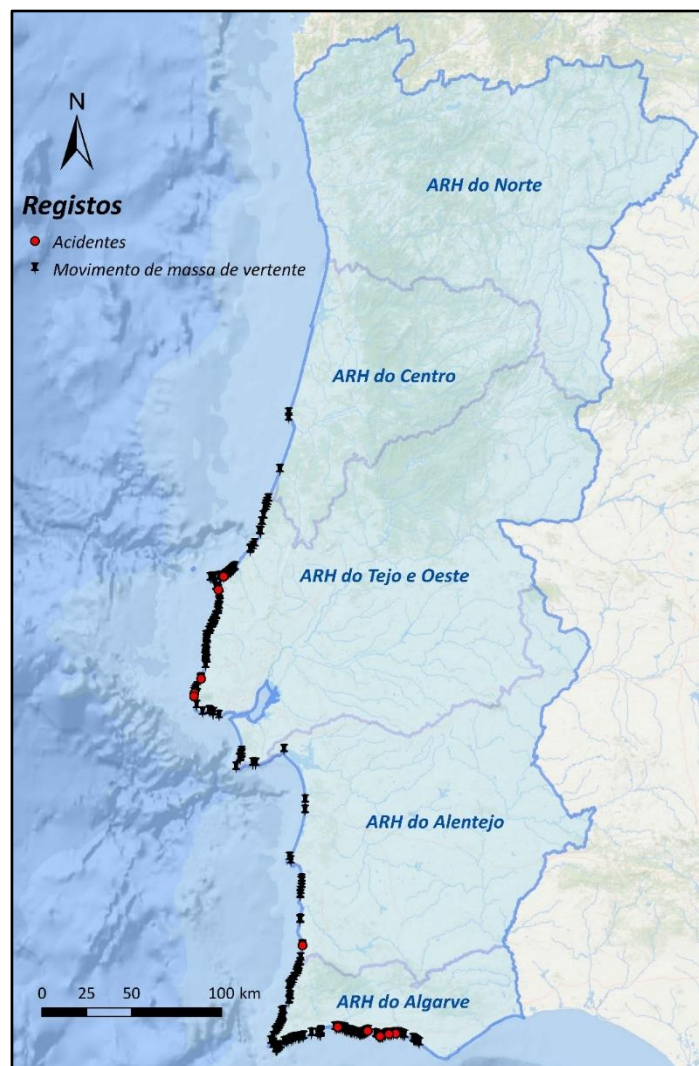
Figura 4.9 – Distribuição espacial das ocorrências de movimentos de massa de vertente em arriba e dos respetivos acidentes com pessoas
