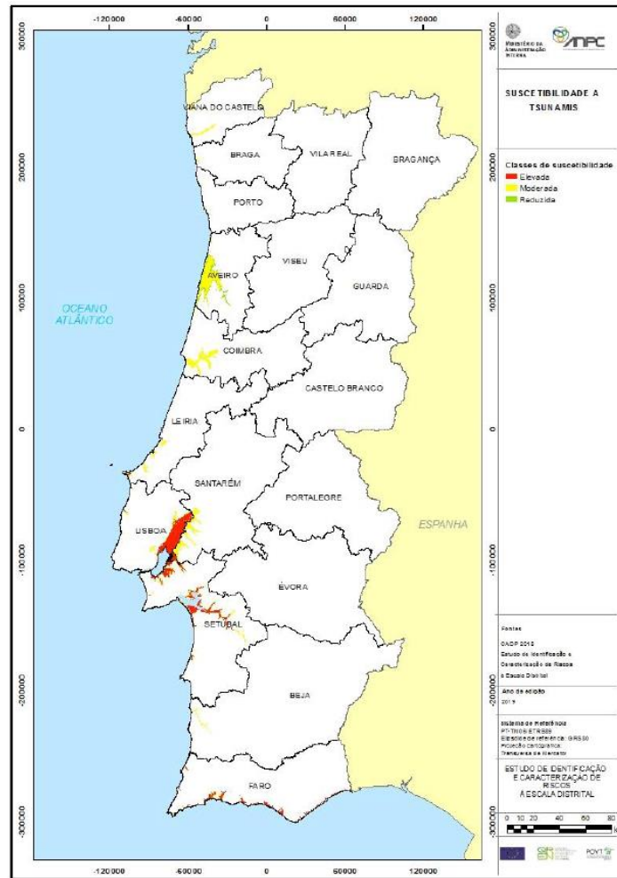
Figura 4.13 – Carta de suscetibilidade a tsunamis (Fonte: Estudos de identificação de riscos à escala distrital – ANPC, 2015)
