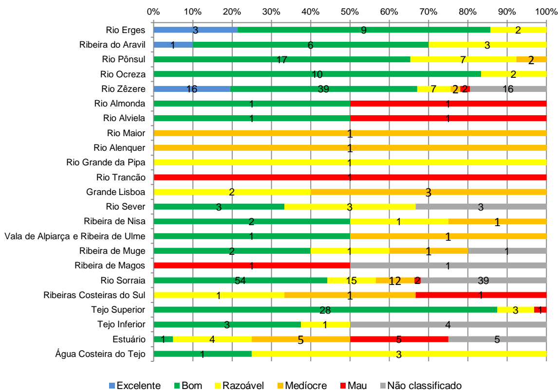
Figura 2.10 – Resultados percentuais do estado das massas de água (MA) por sub-bacia da RH5. Sub-bacias ordenadas segundo um gradiente Norte/Sul, na margem direita e na margem esquerda do rio Tejo.
