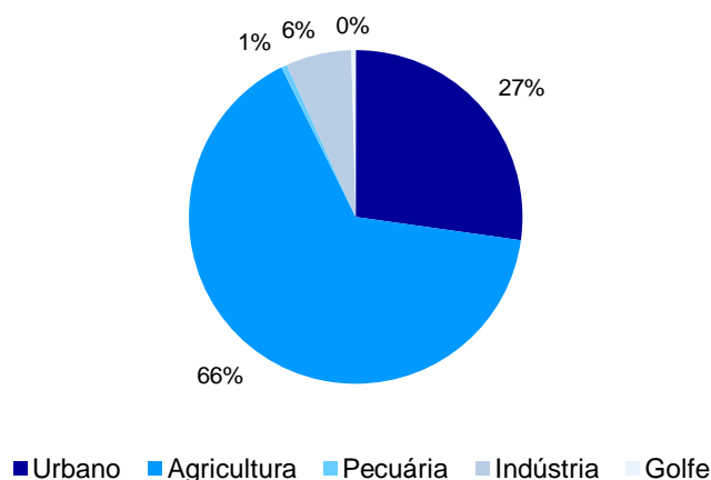
Figura 2.3 – Distribuição das necessidades de água pelos vários usos consumptivos, em ano médio.
