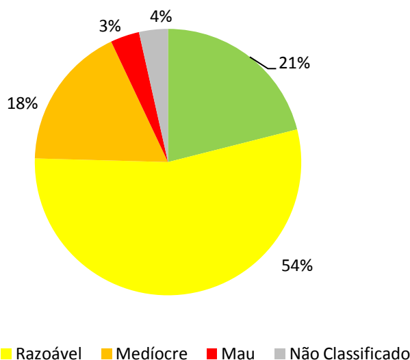
Figura 2.9 – Avaliação do estado ecológico para as massas de Água (MA) naturais da categoria rios, águas de transição e costeiras, e massas de água artificiais (MAA).
