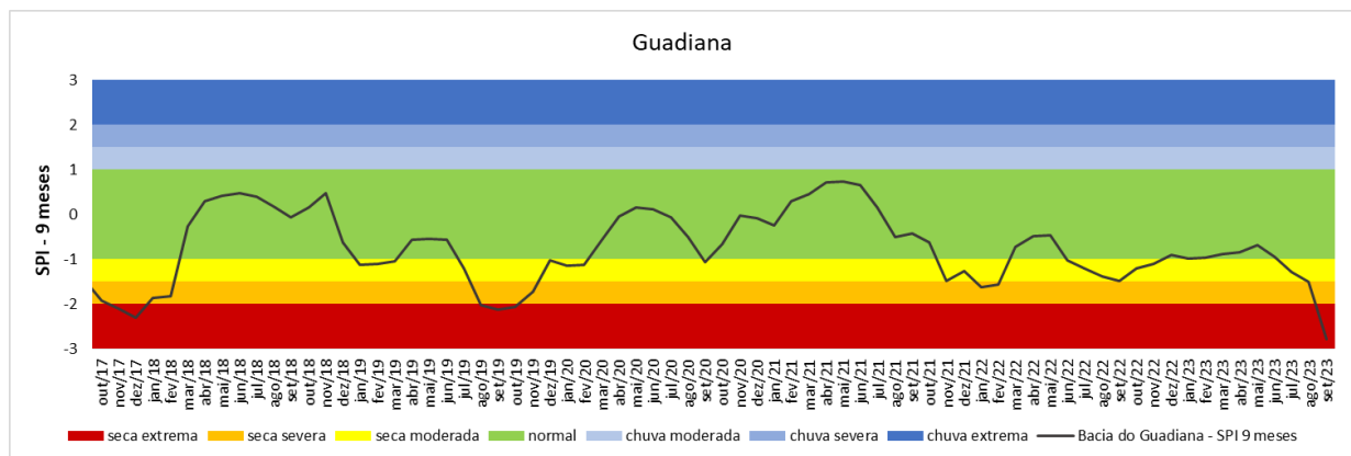
Figura 32 – Índice de seca para a bacia do rio Guadiana, em Portugal.
