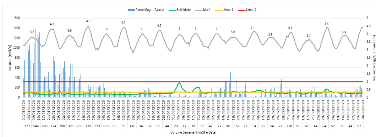
Figura 23 – Variação dos caudais afluentes e da salinidade na seção do rio Tejo à entrada do estuário.
