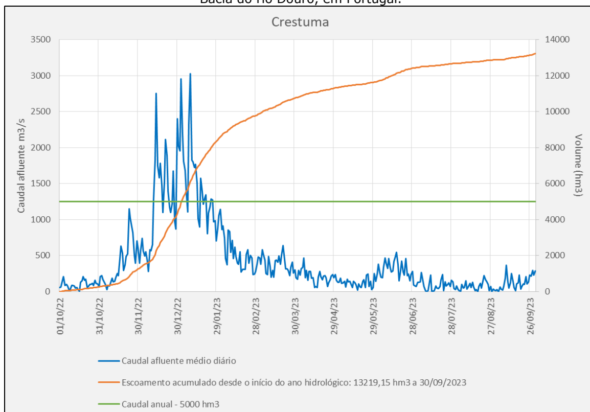
Figura 15 – Caudal médio diário e Volumes acumulados na seção da barragem de Crestuma na Bacia do rio Douro, em Portugal.
