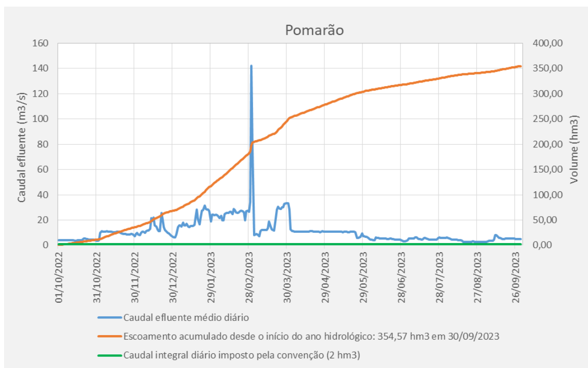
Figura 30 – Caudais médios diários lançados na seção da da estação hidrométrica do Pomarão na Bacia do rio Guadiana, em Portugal.
