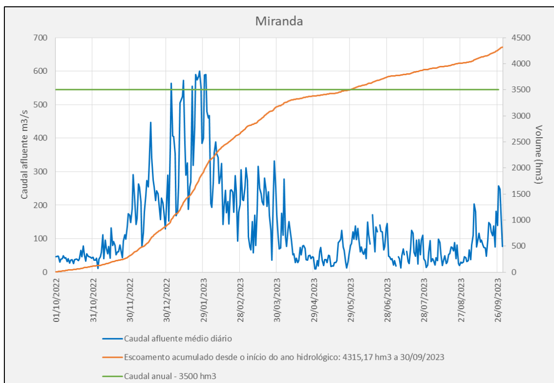
Figura 12 – Caudal médio diário e Volumes acumulados na seção da Barragem de Miranda na bacia do rio Douro, em Portugal.
