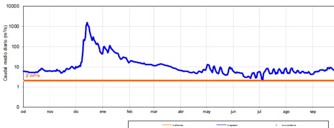
Figura 28 – Caudais médios diários lançados na secção do Açude de Badajoz na bacia do rio Guadiana, em Espanha.
