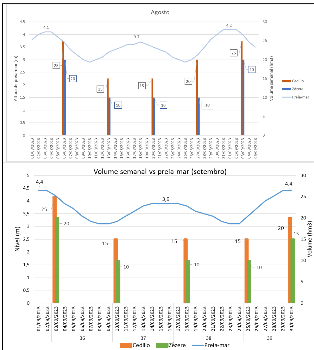
Figura 22 – Volumes semanais solicitados a Espanha para a seção de Cedillo e programados para a seção de Ponte Muge para controlo do avanço da cunha salina à estrada do estuário do Tejo.
