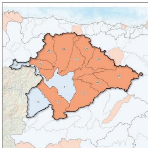
Figura 16 – Índice de seca para o mês de Setembro para bacia do rio Douro, em Espanha.
