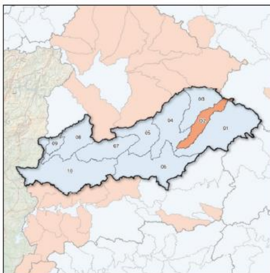
Figura 24 – Índice de seca para o mês de Setembro para bacia do rio Tejo, em Espanha.
