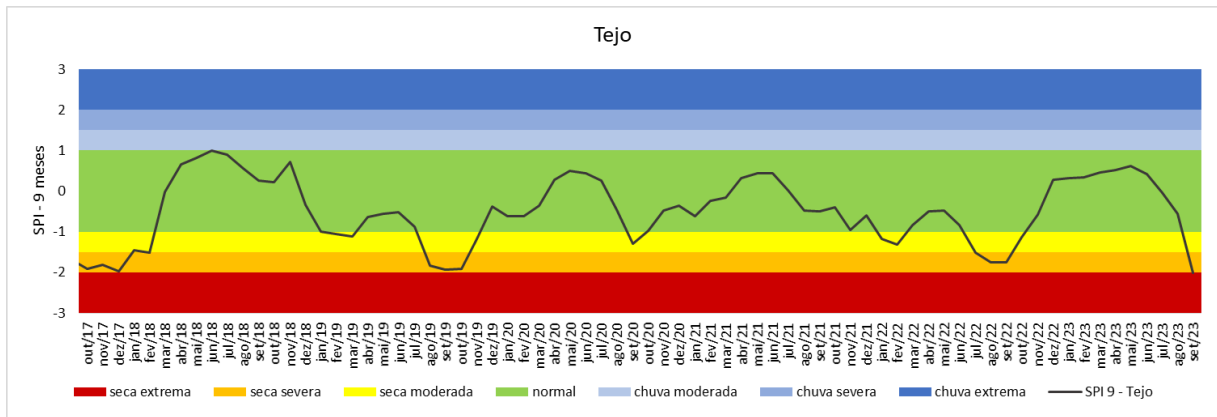
Figura 25 – Índice de seca para a sub-bacia do rio Tejo, em Portugal.
