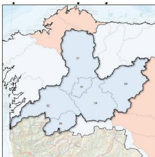
Figura 4 – Índice de seca para o mês de Setembro para bacia do rio Minho, em Espanha.
