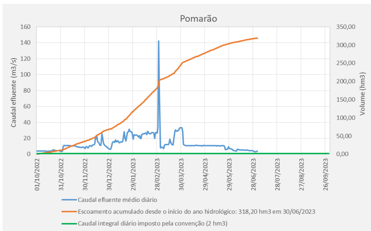
Figura 28 – Caudais médios diários lançados na seção do da estação hidrométrica do Pomarão na Bacia do rio Guadiana, em Portugal.
