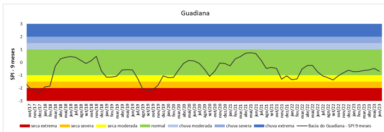
Figura 30 – Índice de seca para a bacia do rio Guadiana, em Portugal.
