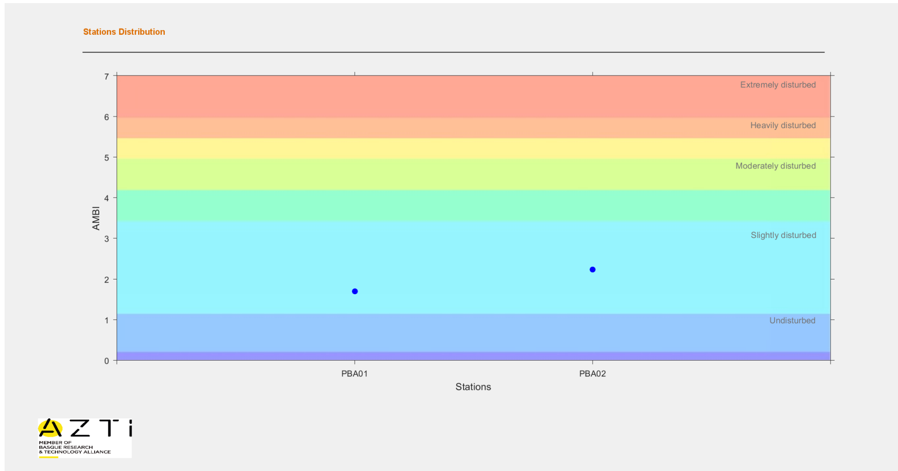
Figura 4.2 - Valor do índice AMBI por local de amostragem (PBA01 – Área de intervenção; PBA02 – Área de controlo) com indicação do grau de perturbação (ligeiramente perturbado).
