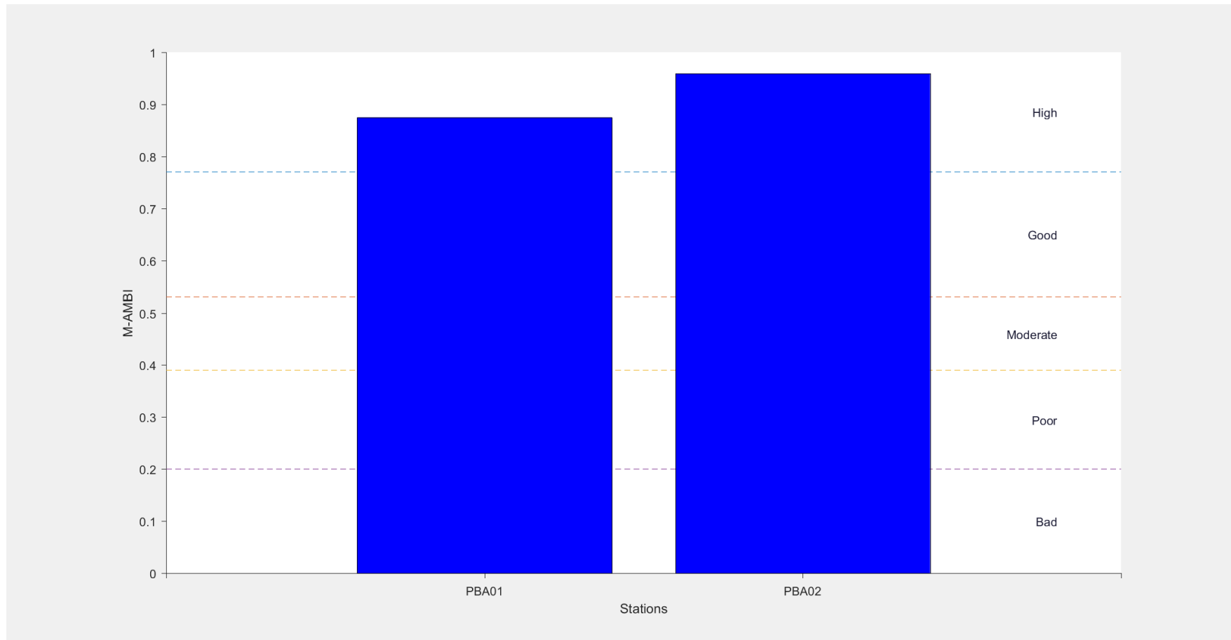
Figura 4.3 - Valor de M-AMBI por local de amostragem (PBA01 – Área de intervenção; PBA02 – Área de controlo) com indicação das classes de qualidade.
