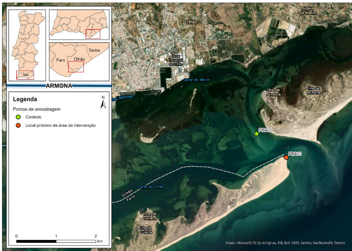
Figura 3.2 - Locais de amostragem de macroinvertebrados bentónicos.
