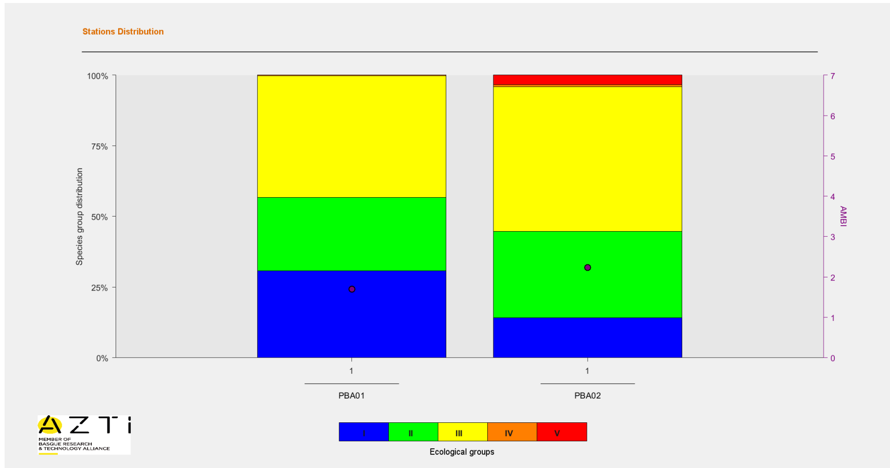
Figura 4.1 - Valor do índice AMBI por local de amostragem (PBA01 – Área de intervenção; PBA02 – Área de controlo) com apresentação da proporção dos grupos ecológicos em função do seu nível de tolerância à perturbação/contaminação (sendo que I são espécies sensíveis e V corresponde a espécie oportunistas de 1ª ordem).
