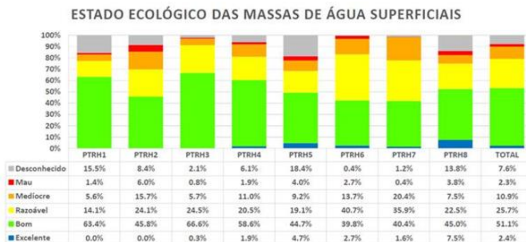
Figura 15- Estado ecológico das massas de águas superficiais obtido no âmbito dos PGRH, publicados em 2013. Fonte: APA, 2013
