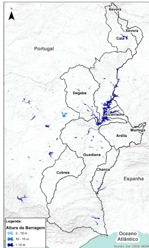
Figura 1 Inventário de barragens e açudes
