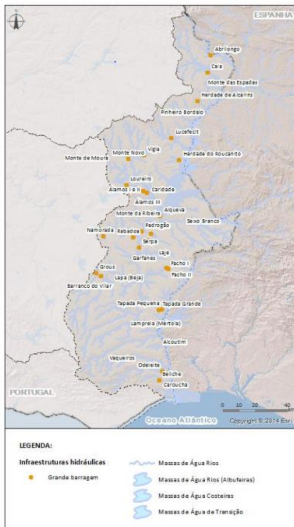
Figura 3 Inventário de Grandes Barragens na RH7 (PGRH 2016-2021)
