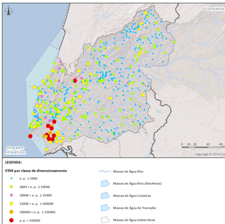
Figura 4 - ETAR por classe de dimensionamento na RH5A.
