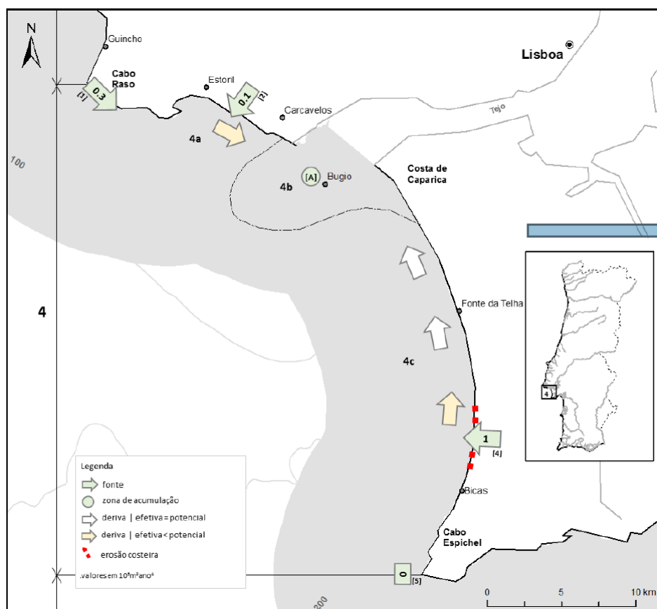
Figura 3 – Célula 4: balanço sedimentar na situação atual (Grupo de Trabalho do Litoral, 2014).
