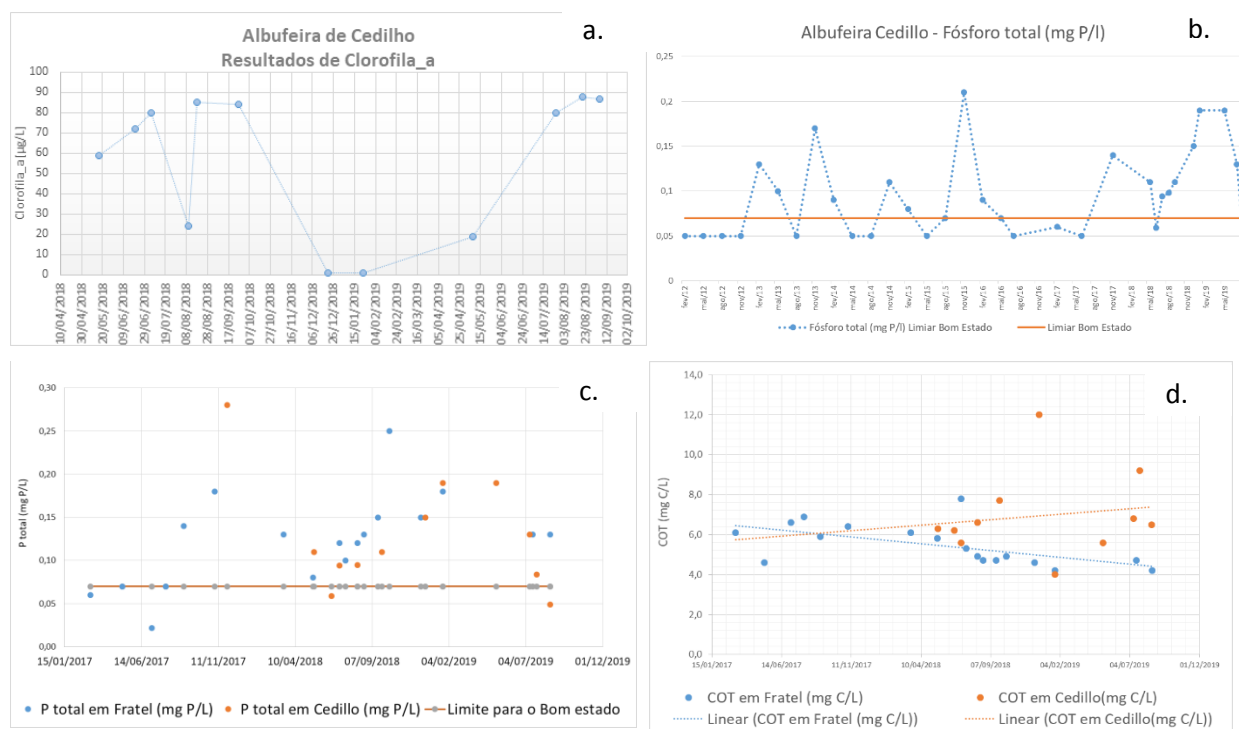
Figura 2 – Variação do Fósforo total, Carbono Orgânico Total (COT) e de Clorofila a nas albufeiras de Cedillo e de Fratel.
