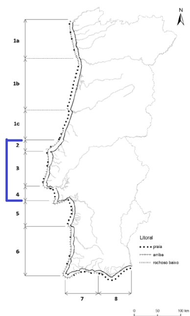
Fig. 1 – Divisão do litoral Português em células sedimentares (GTI, 2014)
