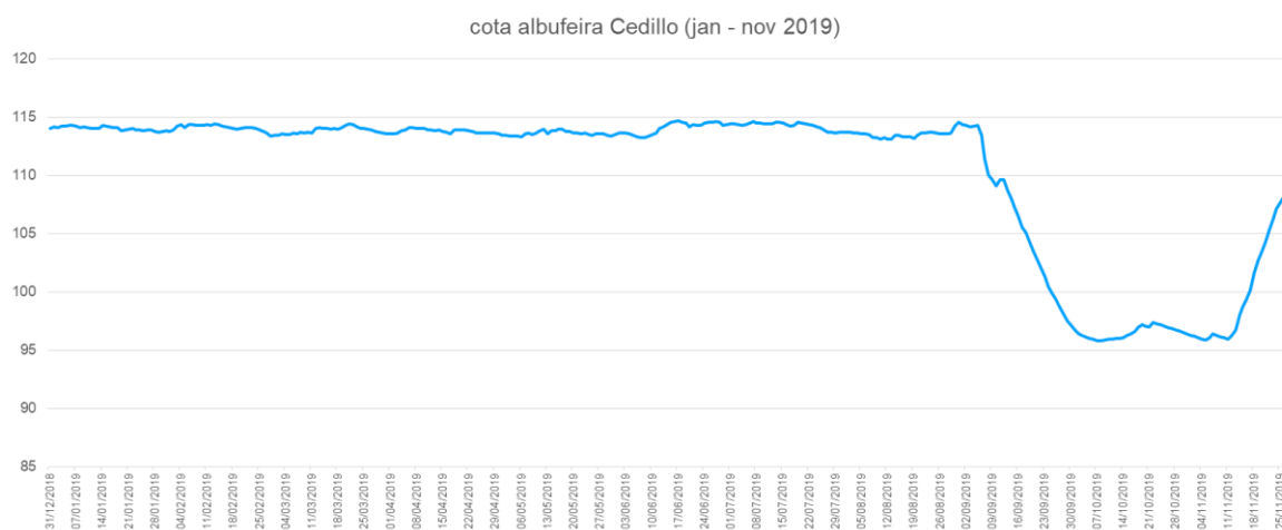
Figura 2 – Cota da albufeira de Cedillo entre janeiro e novembro de 2019.
