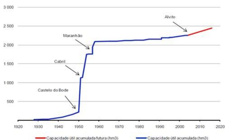
Figura 1 – Evolução da capacidade de armazenamento na RH5
