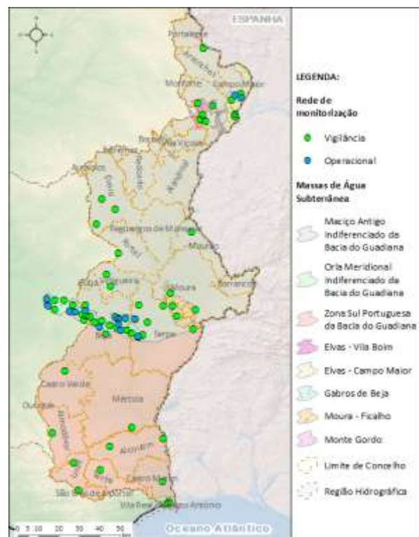
Figura 21- Rede de monitorização do estado quantitativo das águas subterrâneas
