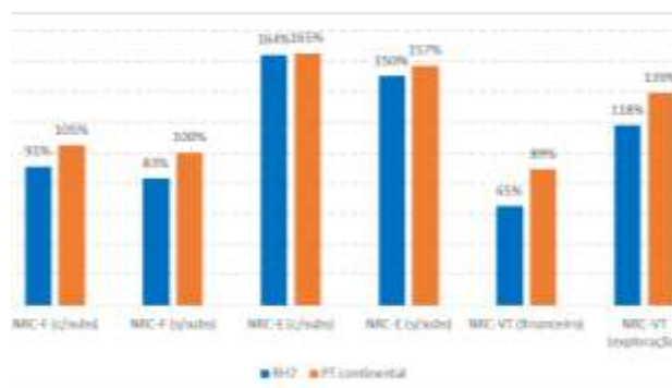
Figura 73 - NRC das entidades gestoras de AA+AR na RH
