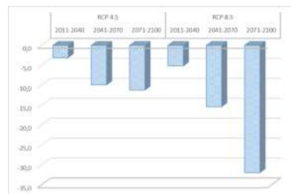
Figura 85 - Variação da recarga média anual para diferentes horizontes temporais na RH (%)
