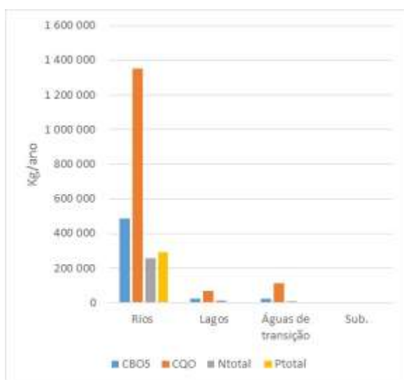
Figura 14 - Cargas rejeitadas pelos sistemas urbanos de drenagem e tratamento de águas residuais urbanas
