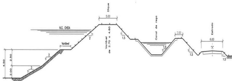
Figura 5 – Perfil do dique lateral e canal
