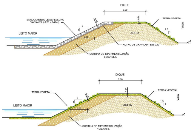
Figura 3 – constituição dos diques de proteção
