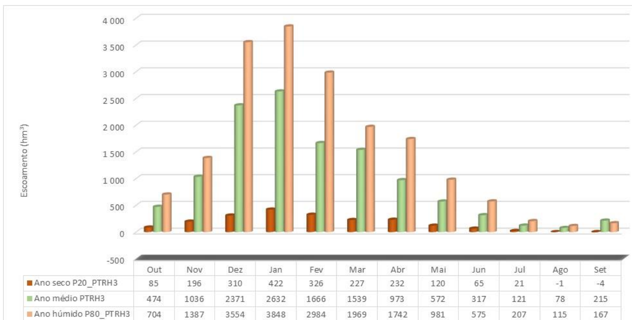
Figura 1.15 – Escoamento em regime modificado mensal para os anos húmido, médio e seco na RH, para o período de referência 1989-2015
