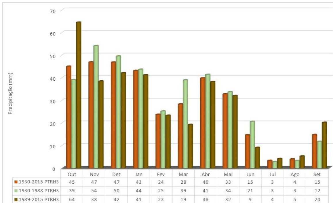
Figura 1.5 – Precipitação média mensal para o ano seco nos três períodos de análise (1930-2015, 1930-1989 e 1989-2015) na RH
