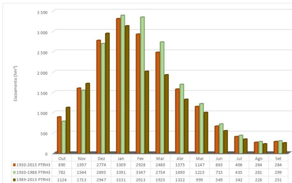
Figura 1.13 – Escoamento médio mensal para o ano médio nos três períodos de análise (1930-2015, 1930-1988 e 1989-2015) na RH
