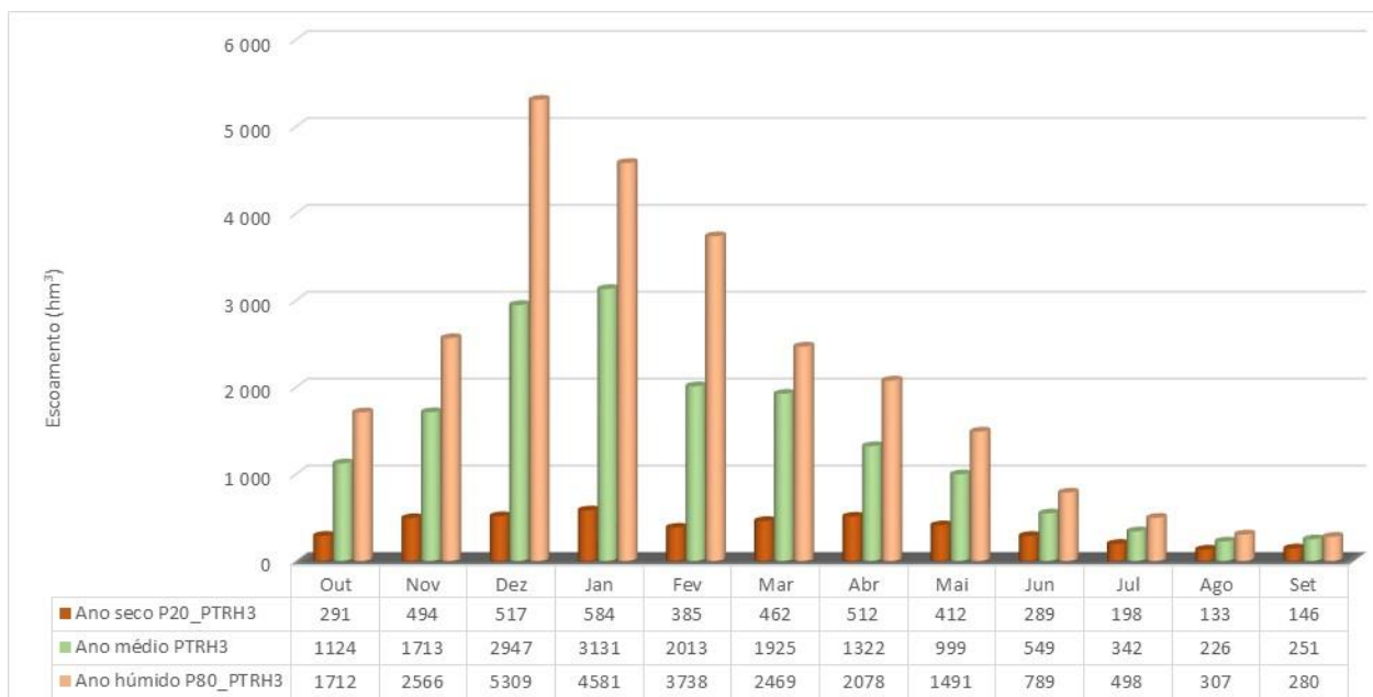
Figura 1.11 – Escoamento médio mensal para os anos húmido, médio e seco para o período de 1989-2015, na RH
