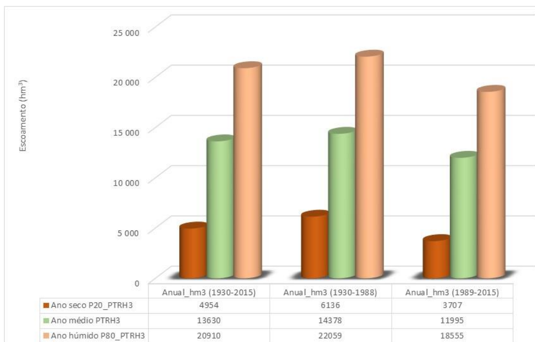
Figura 1.14 – Escoamento anual para o regime modificado para os anos húmido, médio e seco na RH, para os três períodos de referência
