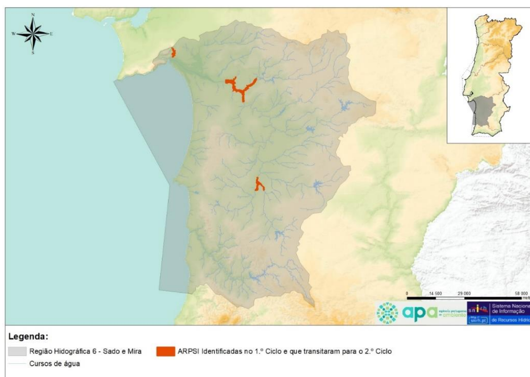
Figura 3.9 - ARPSI identificadas na RH6 (Fonte: PGRI RH6, 2023)
