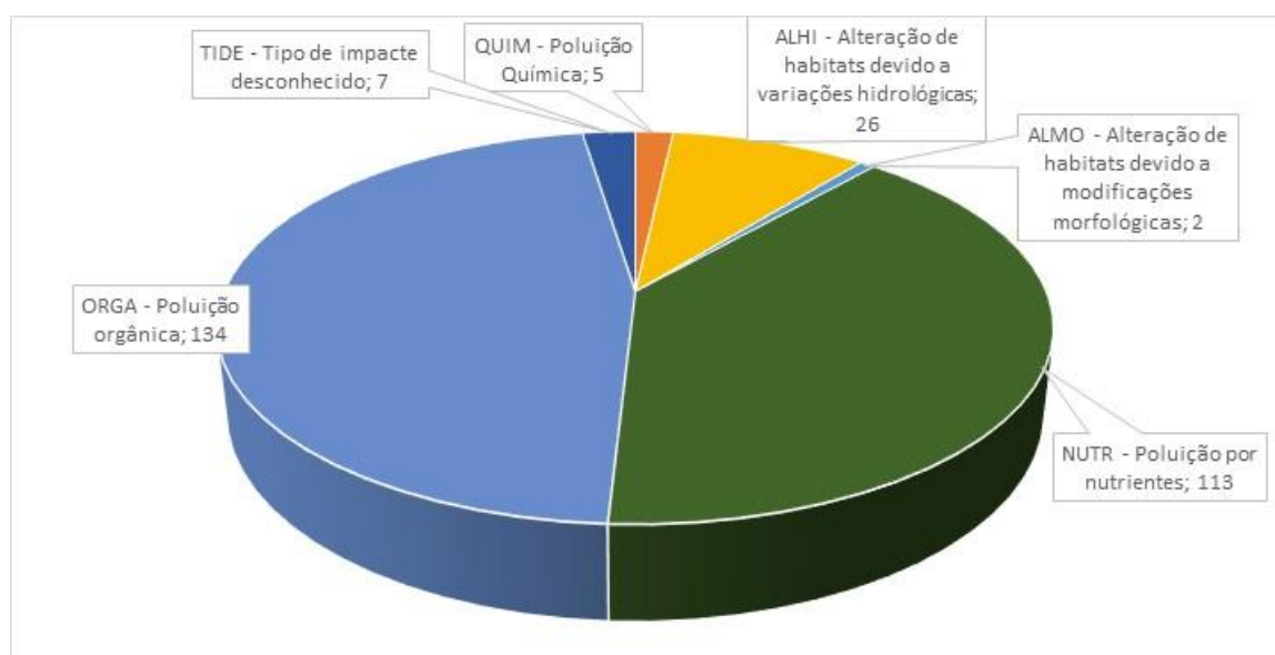
Figura 3.2 - Número de massas de água superficiais associadas a cada tipo de impacto (Fonte: PGRH RH6, 2023)
