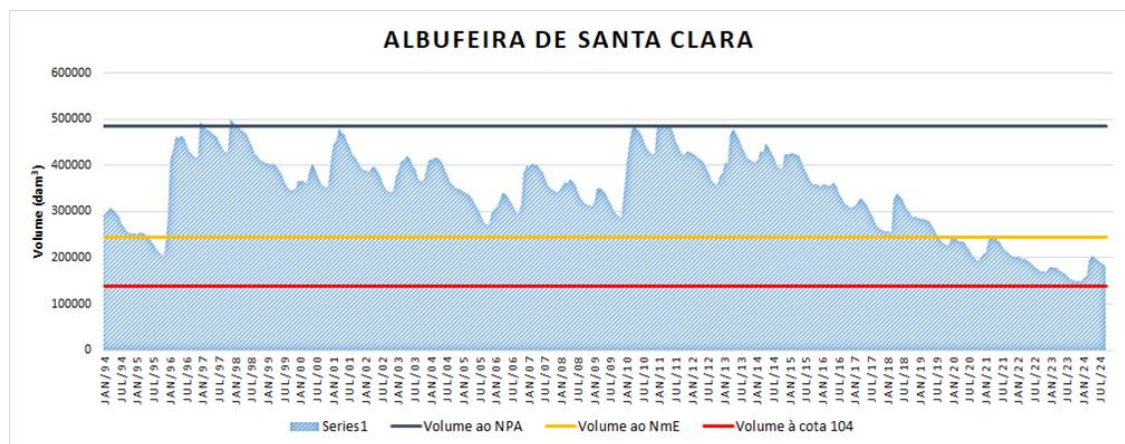
Figura 21 - Evolução dos volumes armazenados na albufeira de Santa Clara (31/01/1994 a 30/09/2024) (Fonte: APA)
