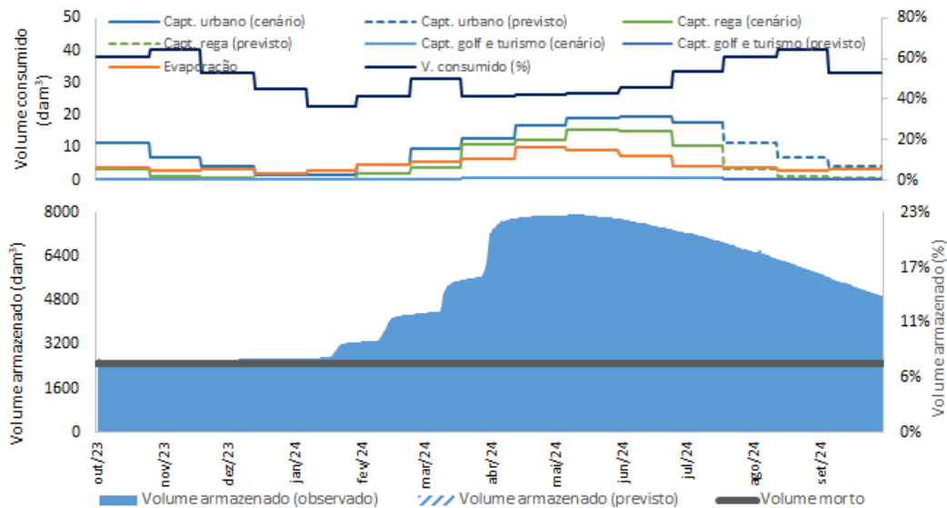
Figura 20- Evolução prevista dos volumes armazenados na albufeira da Bravura considerando a estimativa dos consumos e evaporação até setembro de 2024 (Cenário sem precipitação significativa até ao final do ano) (Fonte: APA)
