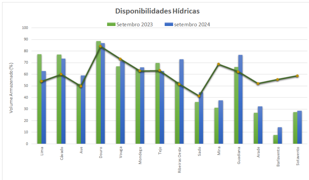
Figura 13 - Percentagem de volume total armazenado por bacia hidrográfica, em 3º de setembro de 2023 e de 2024 (Fonte: APA).
