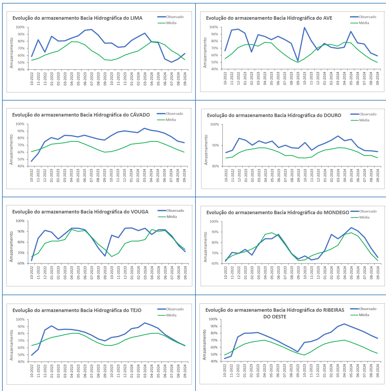
Figura 14 - Evolução do armazenamento desde outubro de 2022 até 30 de setembro de 2024, comparativamente à média (1990/91 a 2019/20) (Fonte: APA)
