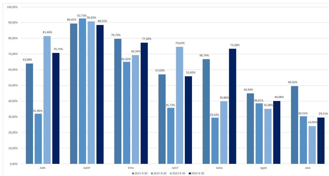
Figura 30 - Volume total armazenado (valores médios) a 30/09 nas albufeiras usadas pelas empresas do grupo AdP para abastecimento público – evolução entre 2021 e 2024 (Fonte: AdP)
