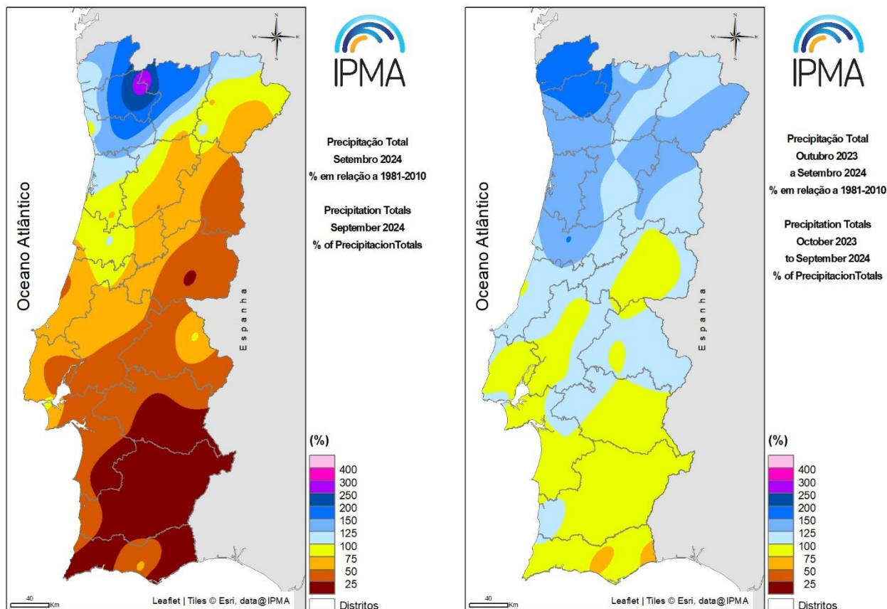
Figura 7 - Distribuição espacial da precipitação (em percentagem) em setembro 2024 (esquerda) e no ano hidrológico 2023/2024 (direita) (Fonte: IPMA)
