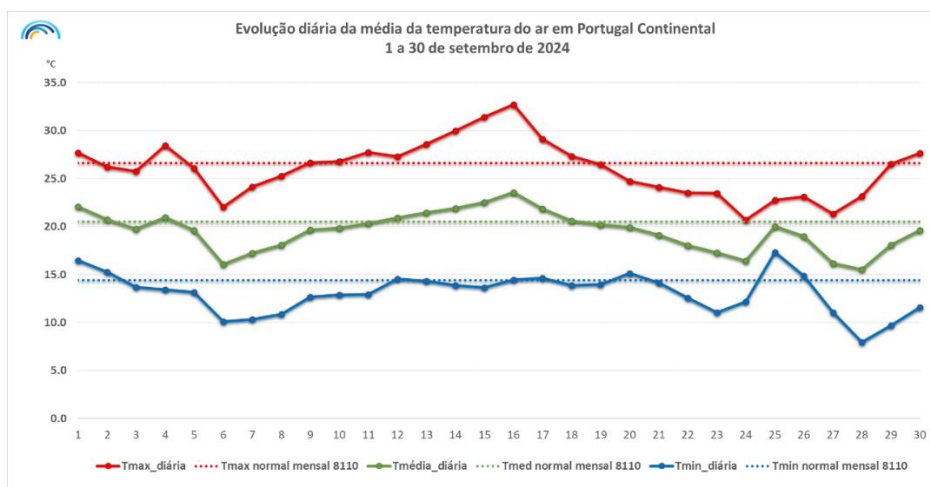
Figura 3 - Evolução diária da temperatura do ar de 1 a 30 de setembro de 2024 em Portugal continental (Fonte: IPMA)
