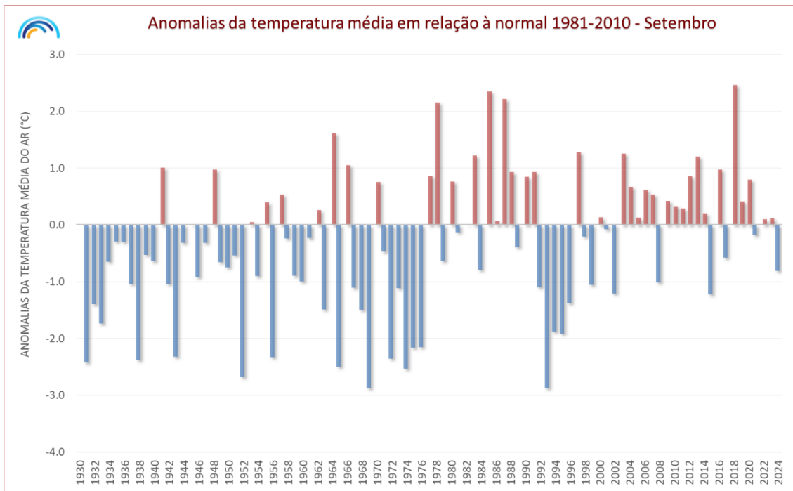
Figura 2 - Anomalias da temperatura média do ar no mês de setembro, em Portugal continental, em relação aos valores médios no período 1981-2000 (Fonte: IPMA)
