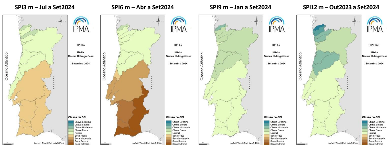
Figura 10 - Distribuição espacial do índice SPI nas escalas de 3, 6, 9 e 12 meses no final de setembro 2024
