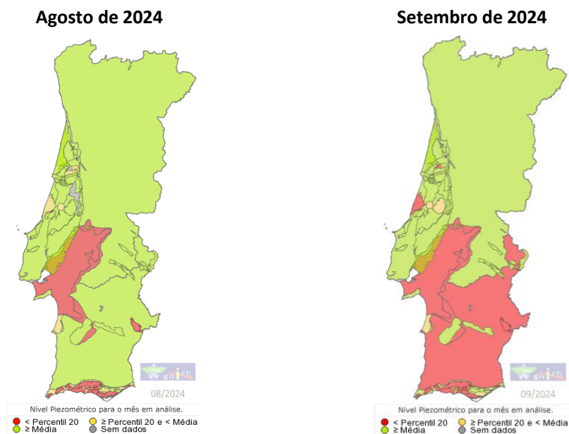
Figura 24 - Evolução das reservas hídricas subterrâneas entre agosto (esquerda) e setembro de 2024 (direita) (Fonte: APA).
