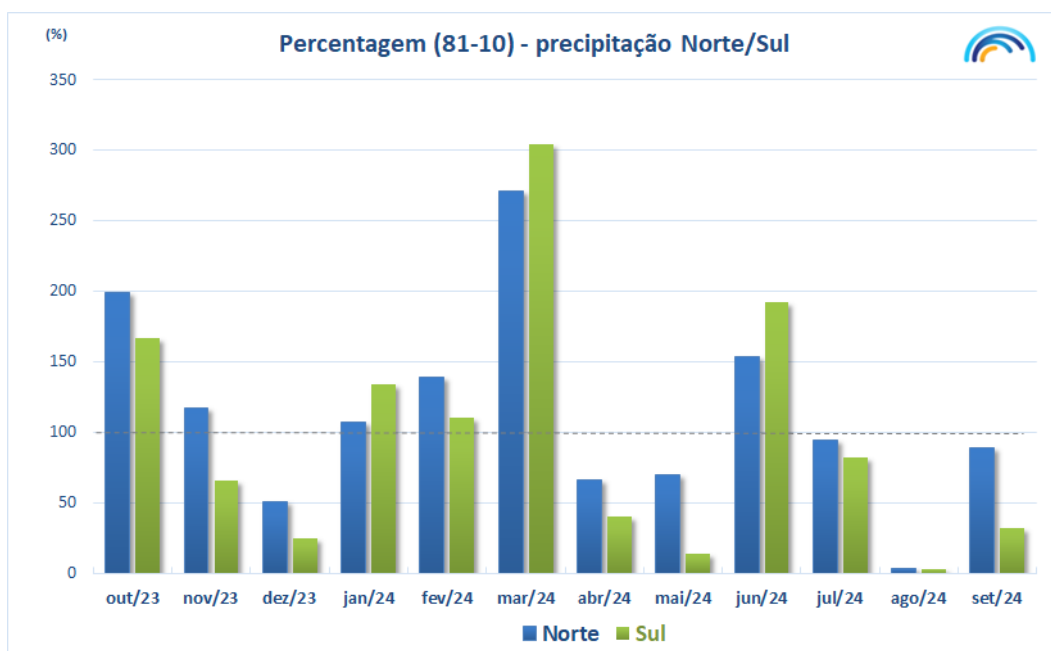
Figura 5 - Percentagem de precipitação em relação ao valor médio 1981-2010 na região a Norte e a Sul do sistema montanhoso Montejunto-Estrela entre outubro 2023 e setembro 2024 (Fonte: IPMA)
