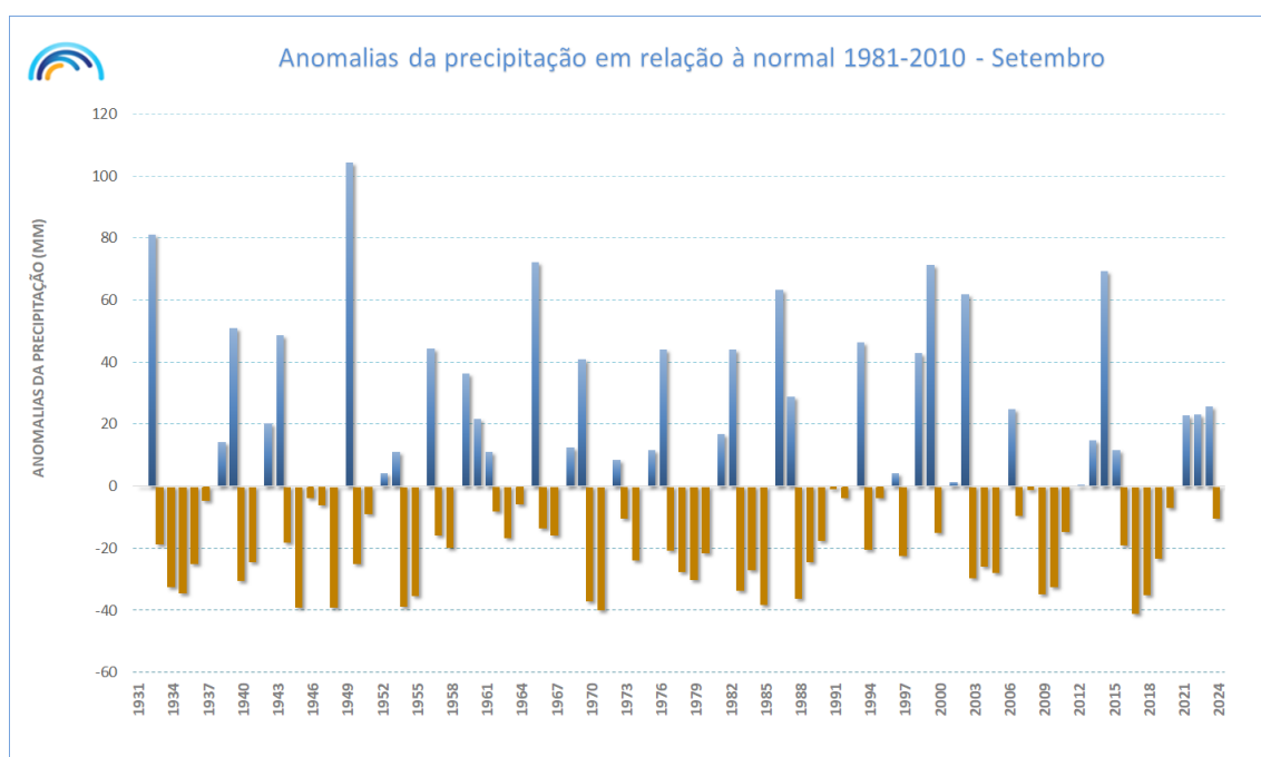
Figura 4 - Anomalias da quantidade de precipitação, no mês de setembro, em Portugal continental, em relação aos valores médios no período 1981-2000 (Fonte: IPMA)
