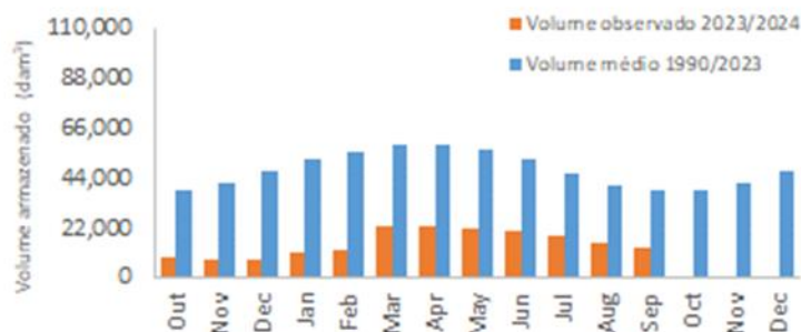
Figura 17- Volumes armazenados desde outubro de 2023 e a média, na albufeira do Monte da Rocha (Fonte: APA)
