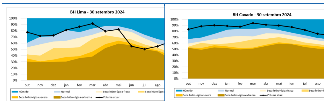
Figura 16 - Nível de armazenamento em setembro de 2024 e os níveis de alerta de seca hidrológica correspondentes a 30 de setembro (Fonte: APA)
