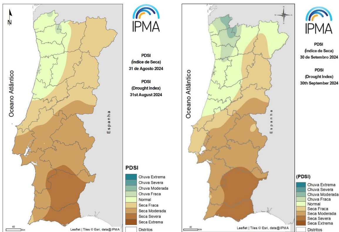
Figura 9 - Distribuição espacial do índice de seca meteorológica a 31 de agosto e a 30 de setembro 2024 (Fonte: IPMA)
