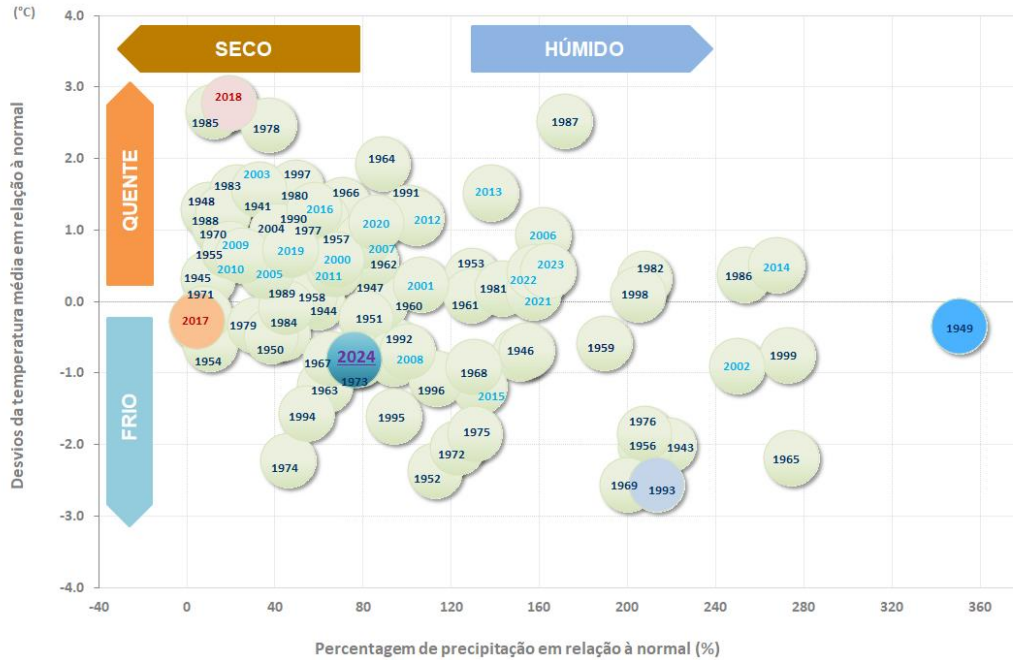
Figura 1 - Desvio da temperatura média do ar e percentagem de precipitação em relação à normal 81-00 no mês de setembro (período 1941 – 2023) (Fonte: IPMA)
