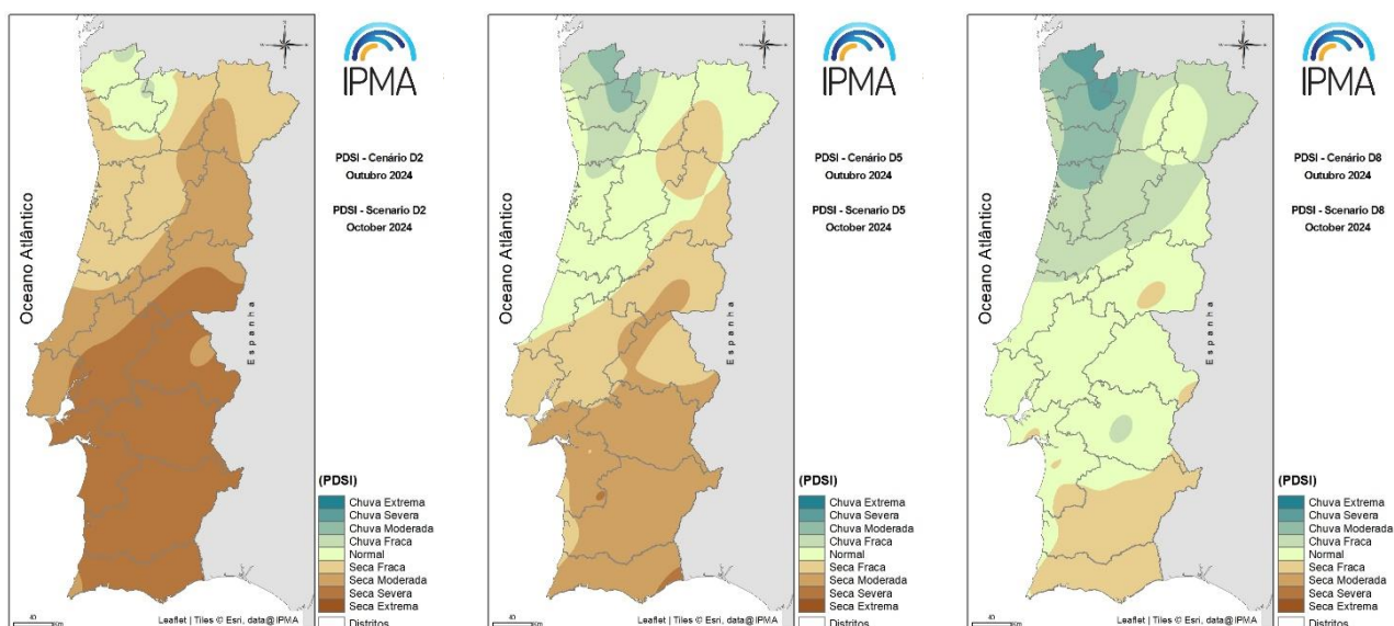
Figura 11 - Distribuição espacial do índice de seca meteorológica PDSI calculado com base em cenários de precipitação para o mês de outubro de 2024 (Fonte: IPMA)
