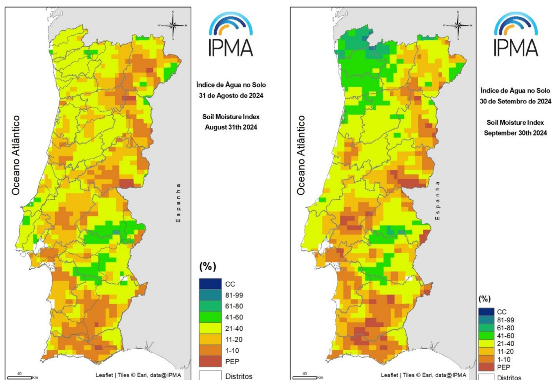
Figura 8 - Percentagem de água no solo (média 0-100 cm profundidade), em relação à capacidade de água utilizável pelas plantas (ECMWF a 31 de agosto e a 30 de setembro de 2024 (Fonte: IPMA)
