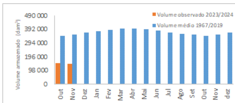
Figura 20 - Volumes armazenados desde outubro de 2023 e a média, na albufeira de Santa Clara (Fonte: APA)
