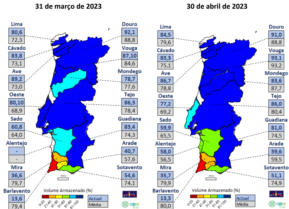
Figura 12 - Situação das albufeiras em março (esquerda) e em abril de 2023 (direita) (Fonte: APA)
