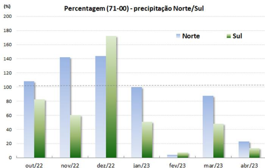
Figura 5 - Percentagem de precipitação em relação ao valor médio 1971-2000 na região a norte e a sul do sistema montanhoso Montejunto-Estrela entre outubro 2022 e abril 2023 (Fonte: IPMA)
