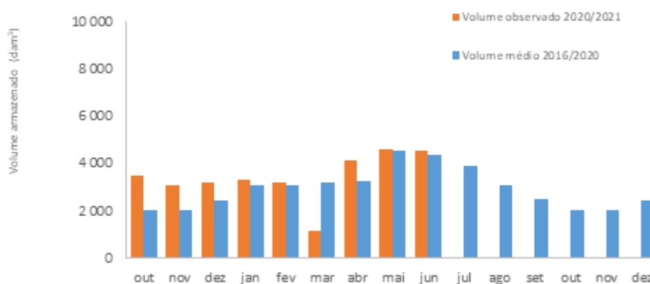
Figura 26 - Comparação entre os volumes armazenados e a média calculada para o período 2016/2020 na albufeira de Fagilde (Fonte: APA)
