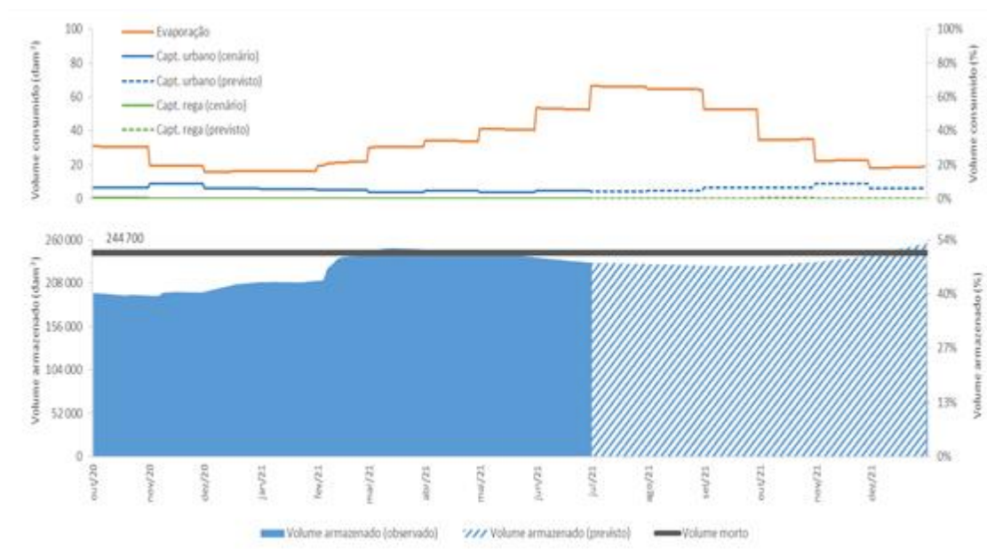
Figura 25. Evolução prevista dos volumes armazenados na albufeira de Santa Clara considerando a estimativa dos consumos e evaporação até dezembro de 2021 (Cenário sem precipitação significativa até ao final do ano) (Fonte: APA).
