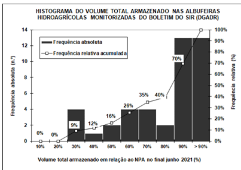
Figura 20. Histograma do volume total armazenado nas albufeiras dos aproveitamentos hidroagrícolas em junho de 2021 (Fonte: DGADR).
