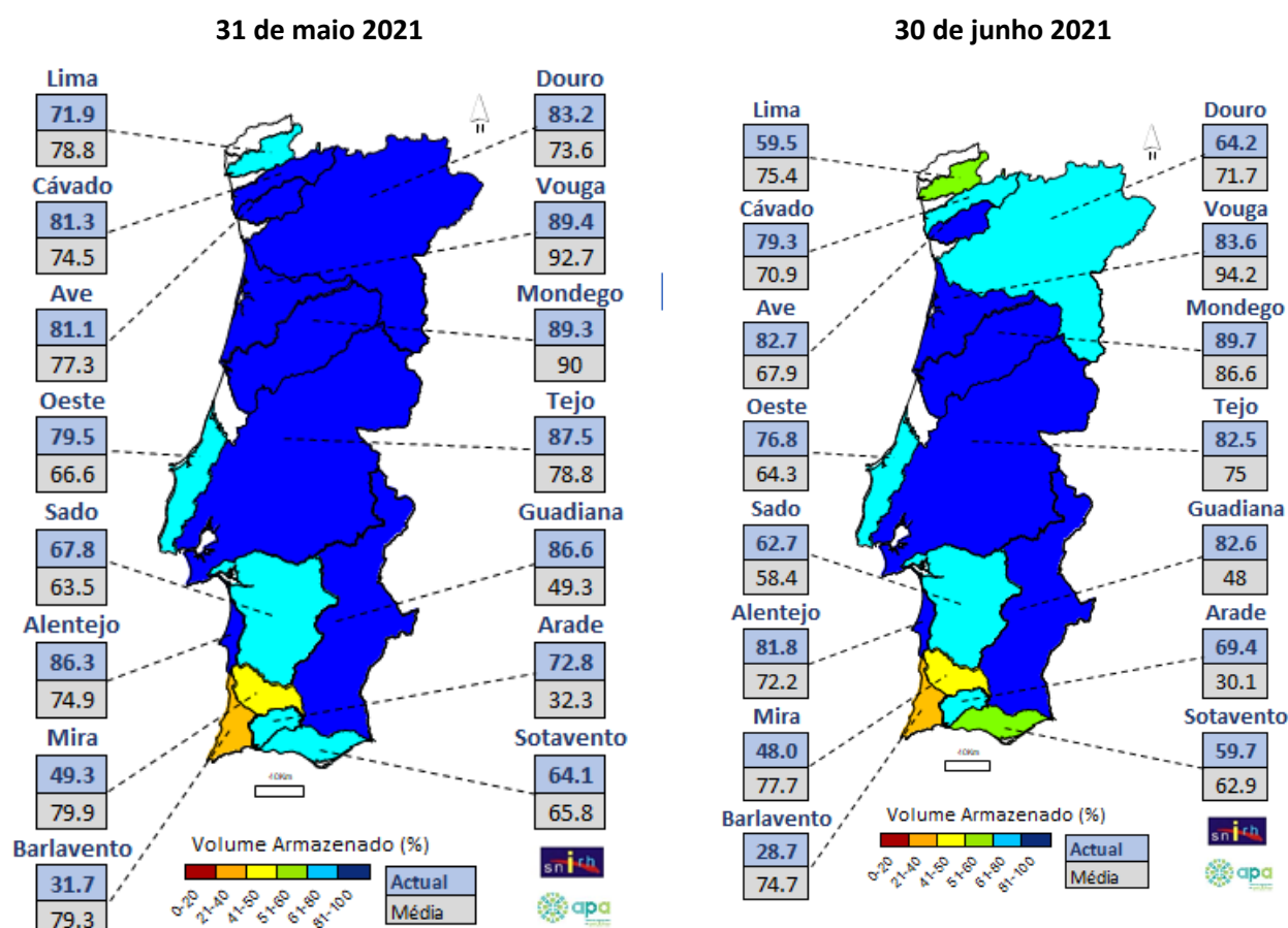
Figura 11. Situação das albufeiras a 31 de maio e de 30 de junho de 2021 (Fonte: APA).
