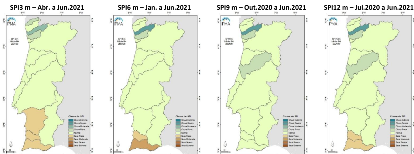
Figura 9. - Distribuição espacial do índice de seca SPI nas escalas de 3, 6, 9 e 12 meses, no final de junho de 2021 (Fonte: IPMA).
