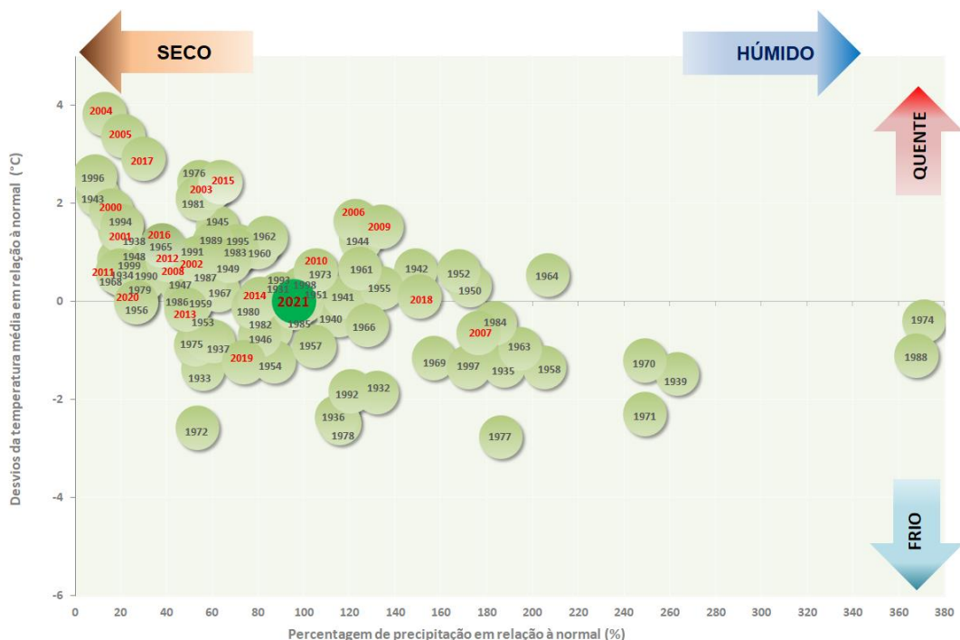
Figura 1. - Desvio da temperatura média do ar e percentagem de precipitação em relação à normal 71-00, mês de junho (período 1931 – 2021) (Fonte: IPMA).
