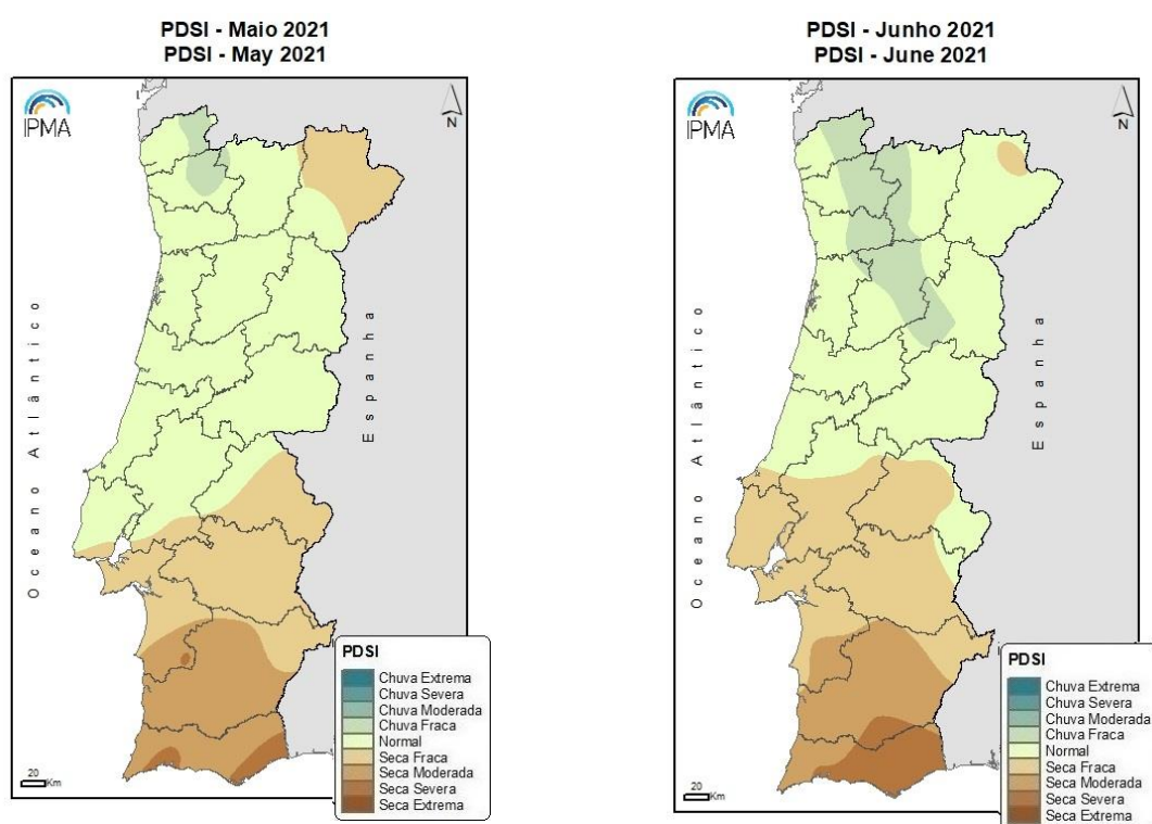
Figura 8. - Distribuição espacial do índice de seca meteorológica a 31 de maio (esquerda) e a 30 de junho de 2021 (direita) (Fonte: IPMA).
