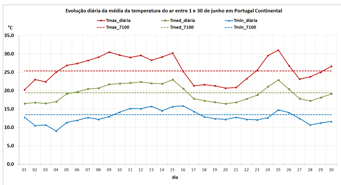
Figura 3. - Evolução diária da temperatura do ar de 1 a 30 de junho de 2021 em Portugal Continental (Fonte: IPMA).
