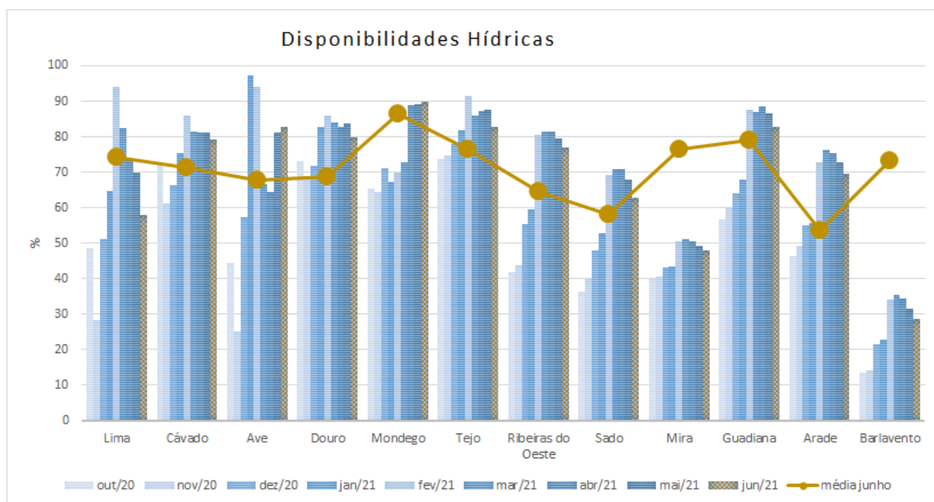
Figura 12 - Percentagem de volume total armazenado por bacia hidrográfica, desde 31 de outubro de 2020 até 30 de junho de 2021, e a média de junho de 2021 (Fonte: APA).
