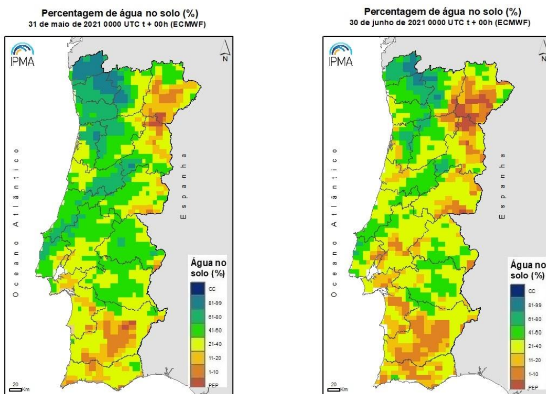
Figura 7. - Percentagem de água no solo (média 0-100 cm profundidade), em relação à capacidade de água utilizável pelas plantas (ECMWF) a 31 de maio de 2021 (lado esquerdo) e a 30 de junho de 2021 (lado direito) (Fonte: IPMA).
