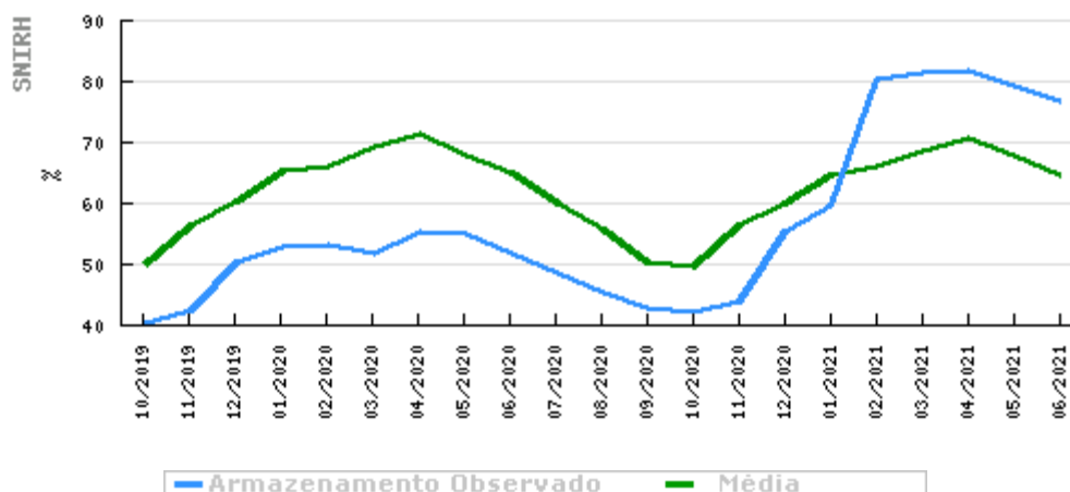
Figura 13. - Evolução dos volumes armazenados na bacia hidrográfica das Ribeiras do Oeste comparativamente à média mensal calculada para o período (1990/91 a 2019/20) (Fonte: APA)
