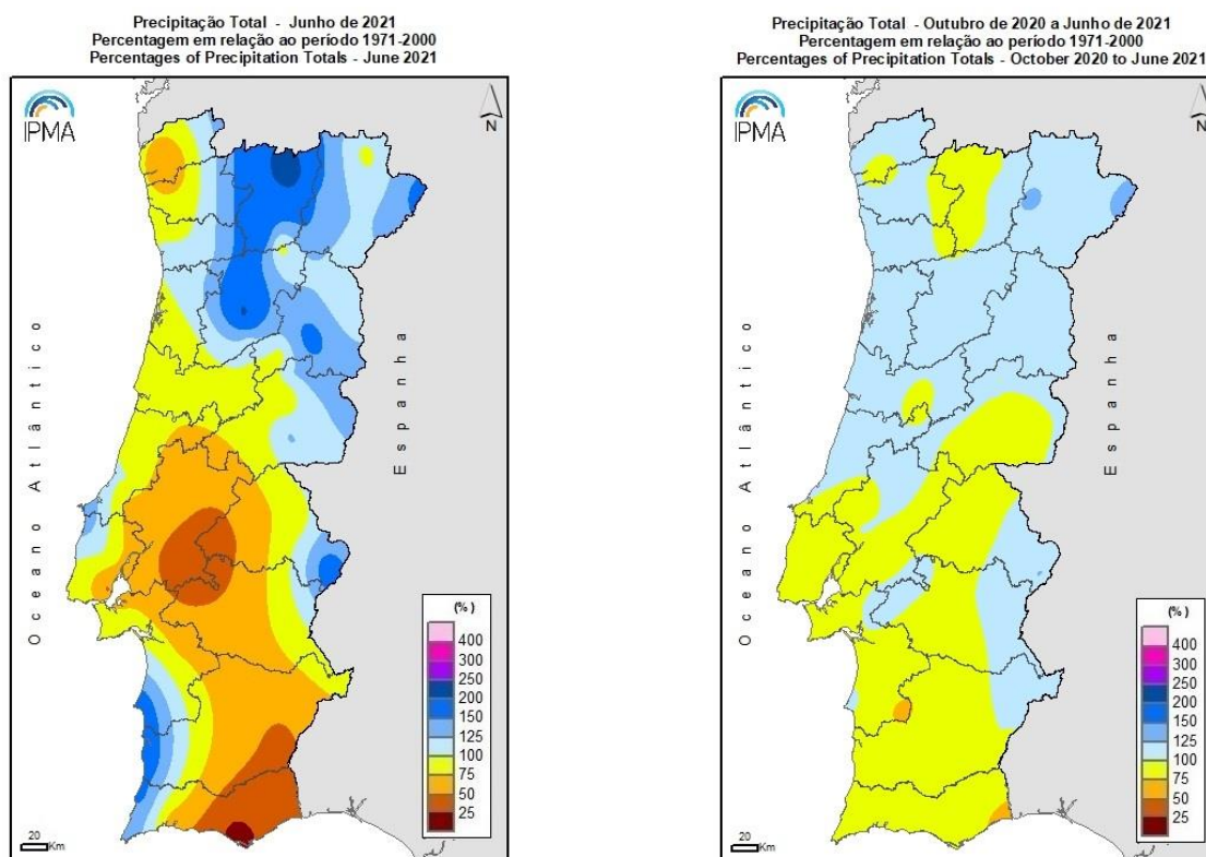
Figura 5. - Distribuição espacial da precipitação (em percentagem) em junho de 2021 (lado esquerdo) e no ano hidrológico 2020/2021 (lado direito) (Fonte: IPMA)
