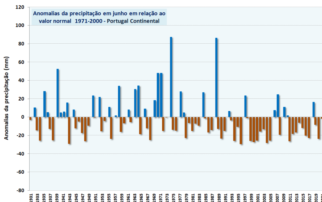
Figura 4.- Anomalias da quantidade de precipitação, no mês de junho, em Portugal continental, em relação aos valores médios no período 1971-2000 (Fonte: IPMA).
