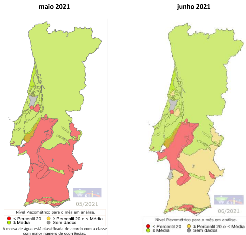
Figura 18 - Evolução das reservas hídricas subterrâneas observadas nos meses de maio e de junho de 2021 (Fonte: APA).
