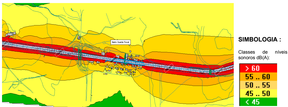
Figura 3 – Exemplo de um mapa de níveis sonoros, na envolvente do bairro da Guarda Fiscal, para o Indicador de Ruído L_n
