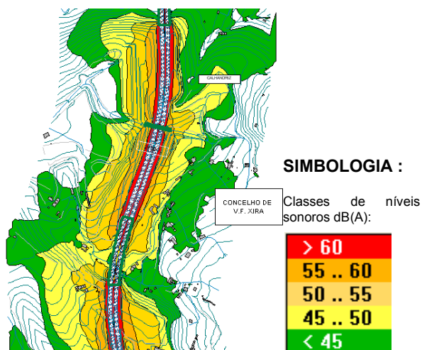
Figura 3 – Exemplo de um mapa de níveis sonoros, na envolvente de Calhandriz, para o Indicador de Ruído L_n
