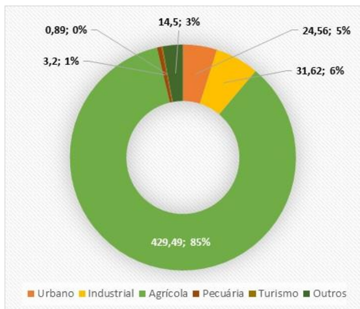
Figura 2.5 - Distribuição dos volumes de água captados pelas principais utilizações consumptivas (hm³)
