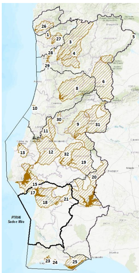
Figura 1.11 – Zonas sensíveis - Revisão de 2020
