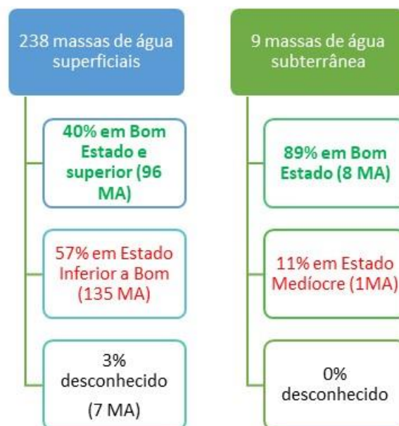
Figura 2.10 - Classificação do estado das massas de água superficiais e subterrâneas no 2.º ciclo de planeamento
