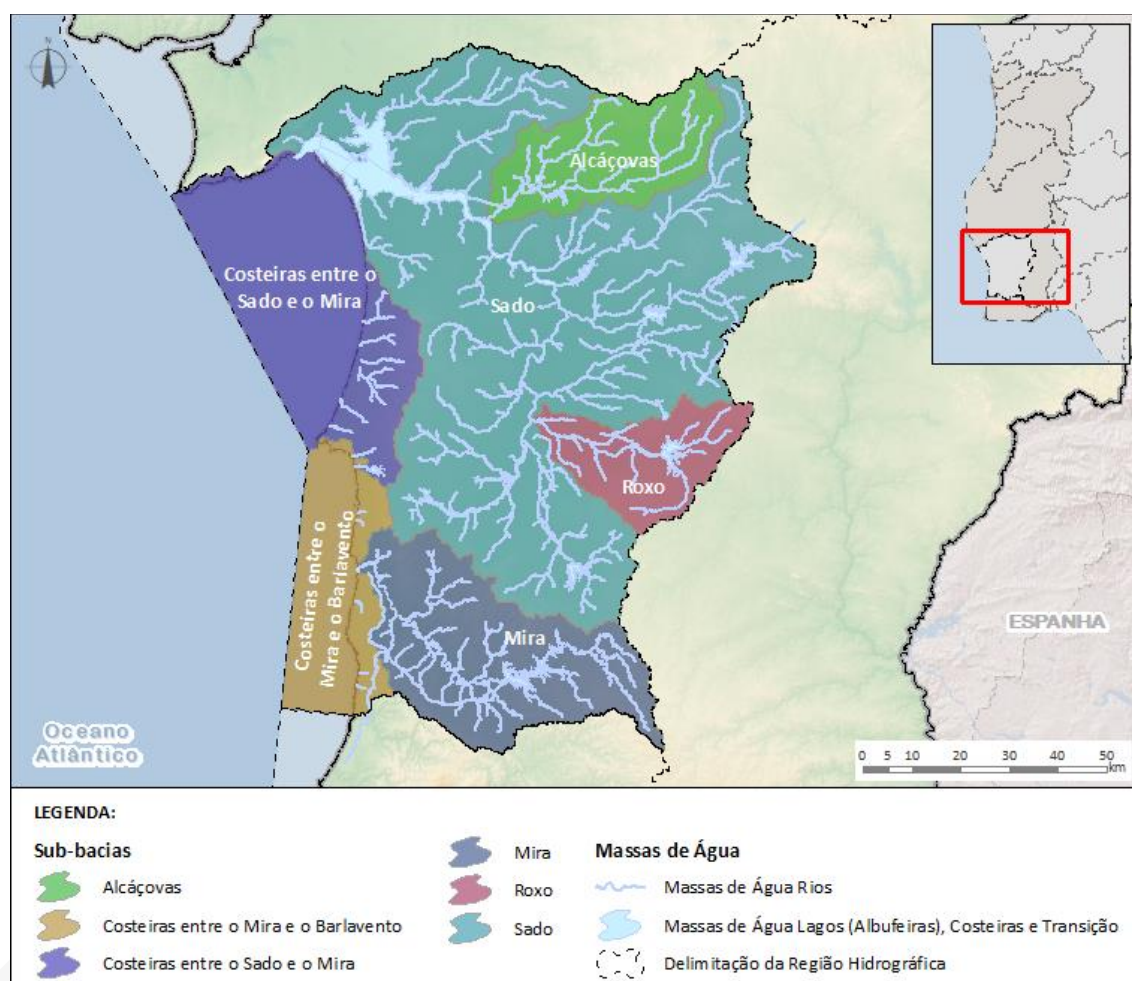
Figura 2.1– Delimitação das sub-bacias identificadas na RH6
