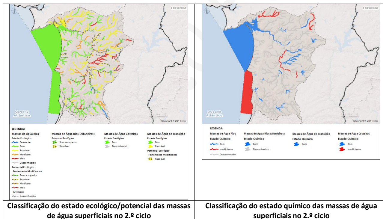
Figura 2.8 – Classificação do estado das massas de águas superficiais
