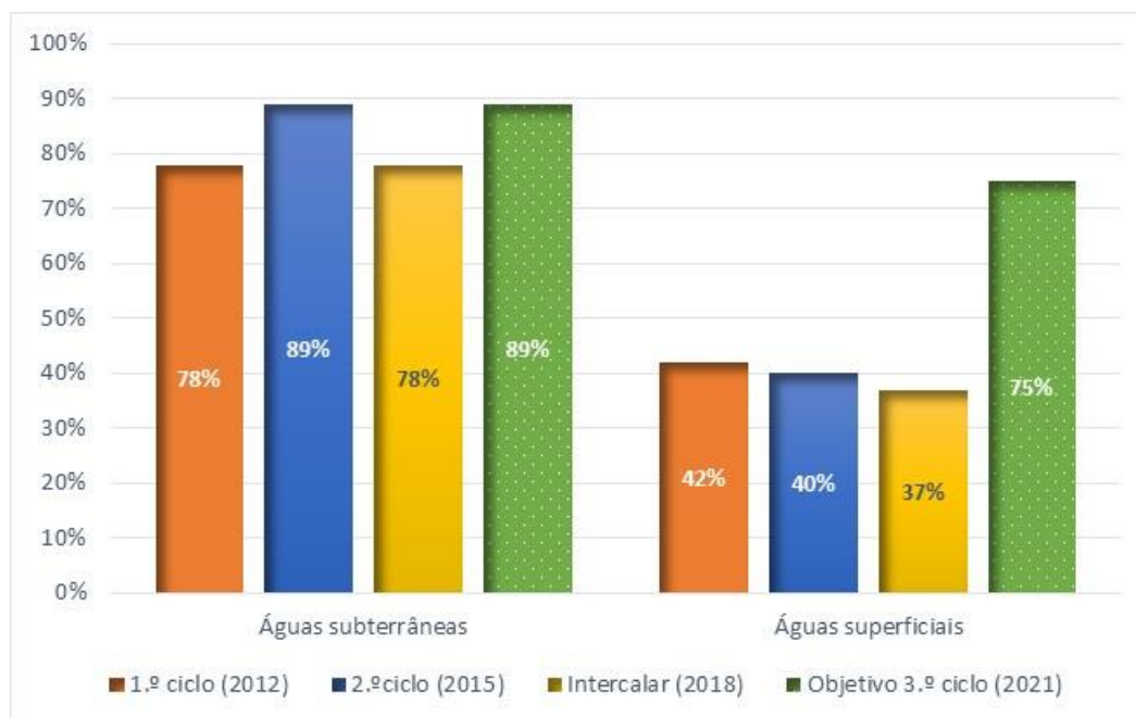
Figura 2.11 – Evolução da classificação das massas de água superficiais e subterrâneas em Bom estado
