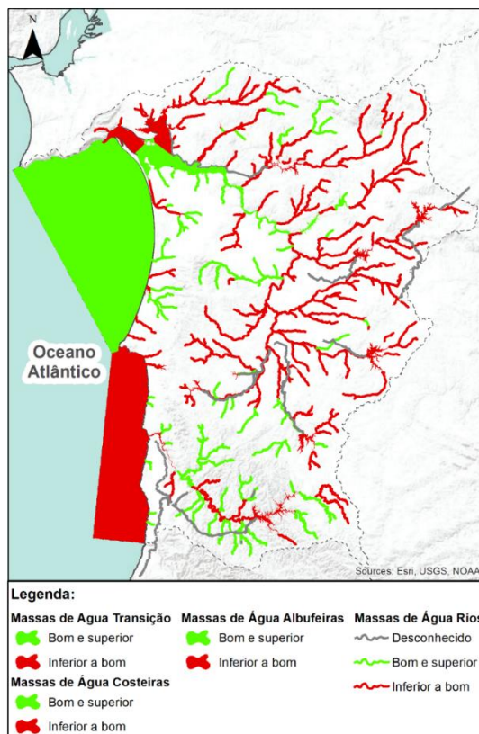
Figura 1 Estado global das massas de água superficiais na RH6 (2016-2021)
