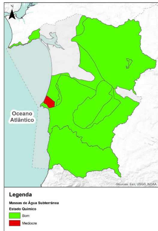
Figura 1 Estado químico das massas de água subterrâneas na RH6 (2016-2021)
