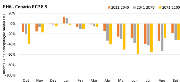
Figura 2 – Anomalia das precipitações médias mensais na RH6 (%), cenário RCP 8.5
