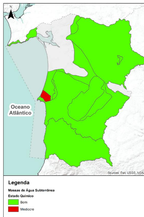
Figura 3 Estado químico das massas de água subterrâneas na RH6 (2016-2021)
