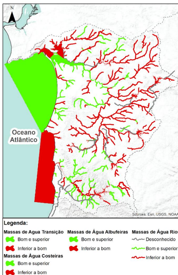
Figura 4 Estado global das massas de água superficiais na RH6 (2016-2021)
