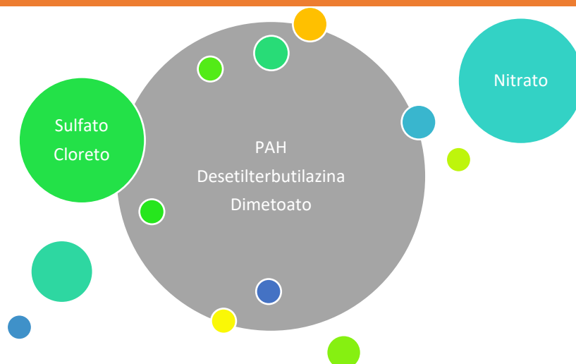
Figura 2 Parâmetros/substâncias submetidos a teste (princípio “ONE OUT ALL OUT”) para avaliação do estado químico das massas de água subterrâneas na RH6 (2018)
