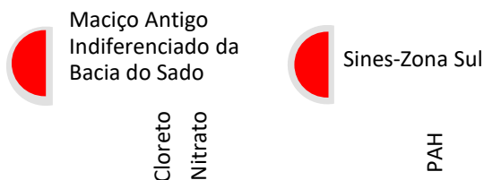
Figura 3 Parâmetros responsáveis pelo estado químico inferior a bom das massas de água subterrâneas na RH6 (2018)
