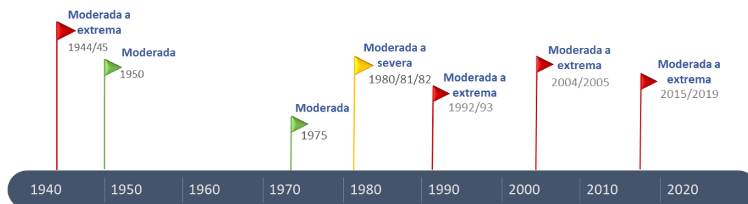
Figura 4 Ocorrência de secas em Portugal continental
