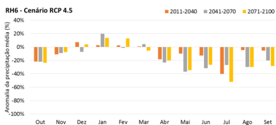
Figura 1 – Anomalia das precipitações médias mensais na RH6 (%), cenário RCP 4.5
