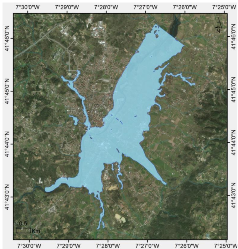
Figura 3. Zona Crítica de Chaves – área inundada para o período de retorno de 100 anos
