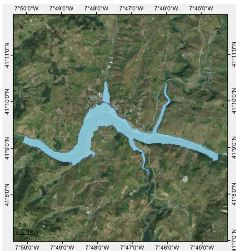
Figura 5. Zona Crítica da Régua – área inundada para o período de retorno de 100 anos
