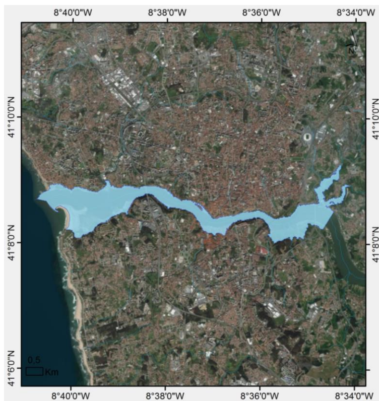
Figura 4. Zona Crítica do Porto/Vila Nova de Gaia – área inundada para o período de retorno de 100 anos
