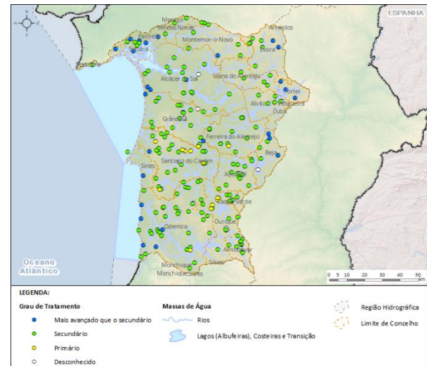
Figura 12 - Pontos de descarga das ETAR públicas urbanas no meio hídrico
