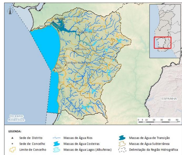
Figura 4 - Delimitação geográfica da região hidrográfica do Sado e Mira (RH6)
