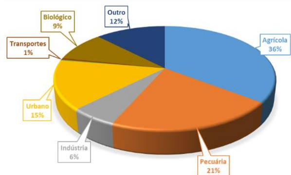
Figura 100 - Setores e subsectores responsáveis pelas pressões significativas nas massas de água superficiais
