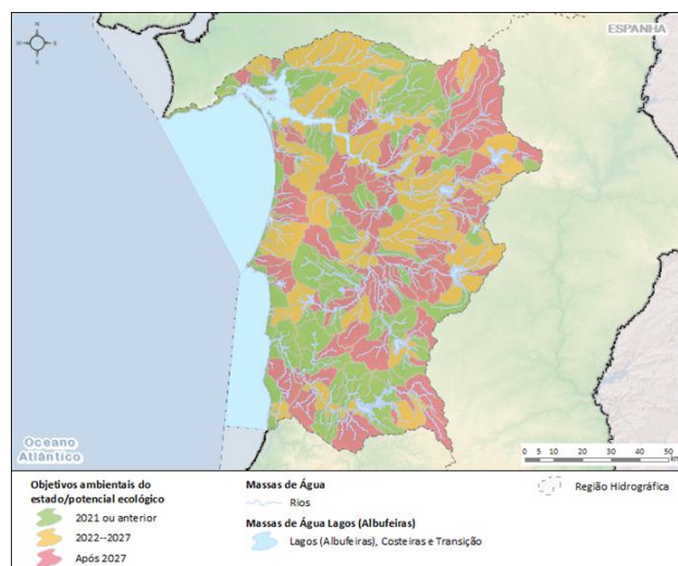
Figura 93 - Objetivos ambientais para as massas de água superficiais – Estado/potencial ecológico
