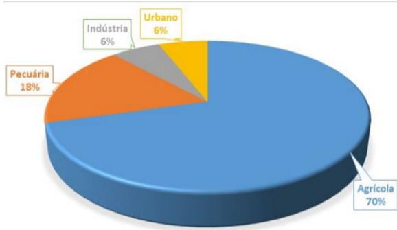
Figura 101 - Setores e subsectores responsáveis pelas pressões significativas nas massas de água subterrâneas
