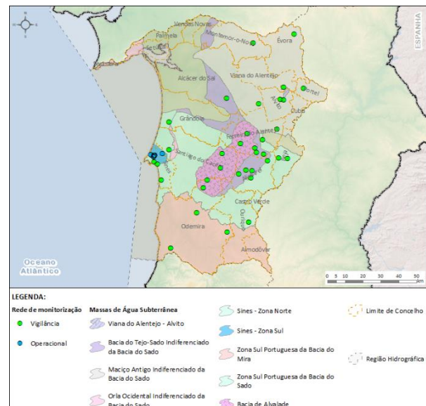
Figura 19 - Rede de monitorização do estado químico das águas subterrâneas
