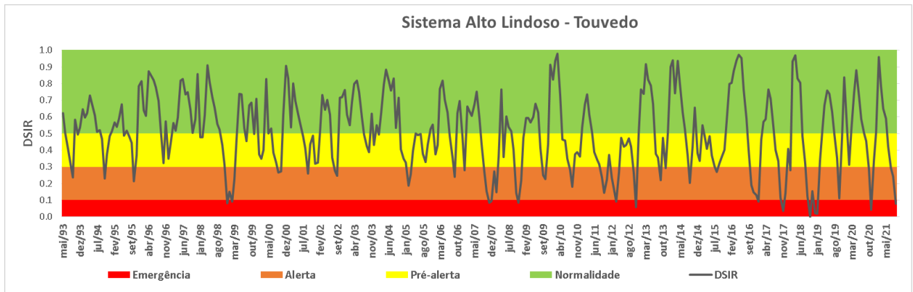
Figura 4.4 – Aplicação do índice Drought State Index for Reservoirs na RH1, sistema Alto Lindoso - Touvedo
