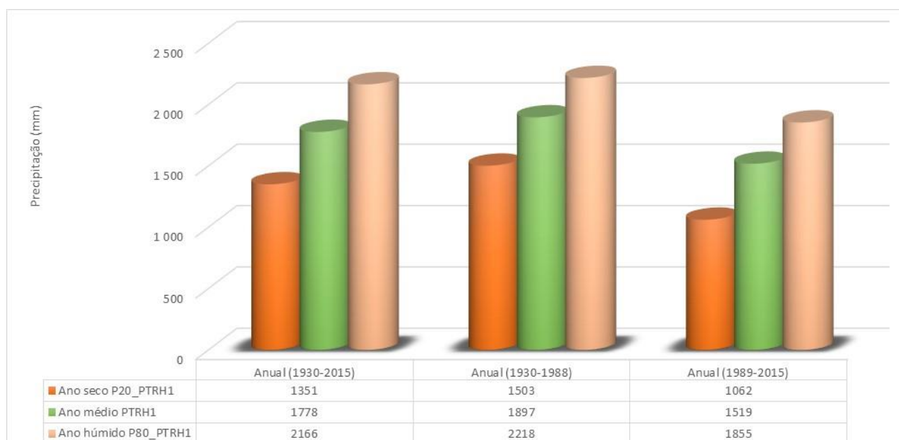
Figura 1.2 – Precipitação média anual para os anos húmido, médio e seco na RH, para os três períodos de referência
