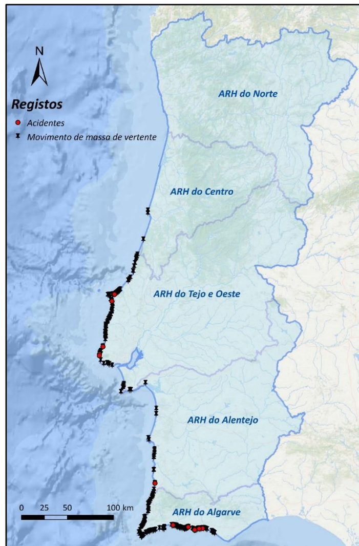
Figura 4.8 – Distribuição espacial das ocorrências de movimentos de massa de vertente em arriba e dos respetivos acidentes com pessoas
