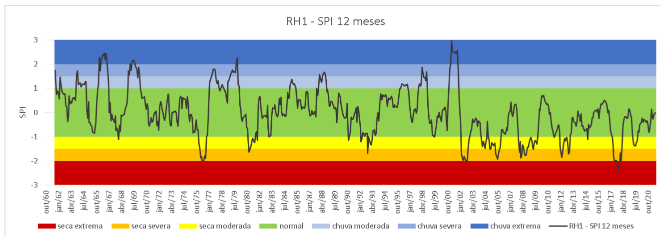
Figura 4.3 – Índice SPI-12 para a Região Hidrográfica Minho e Lima
