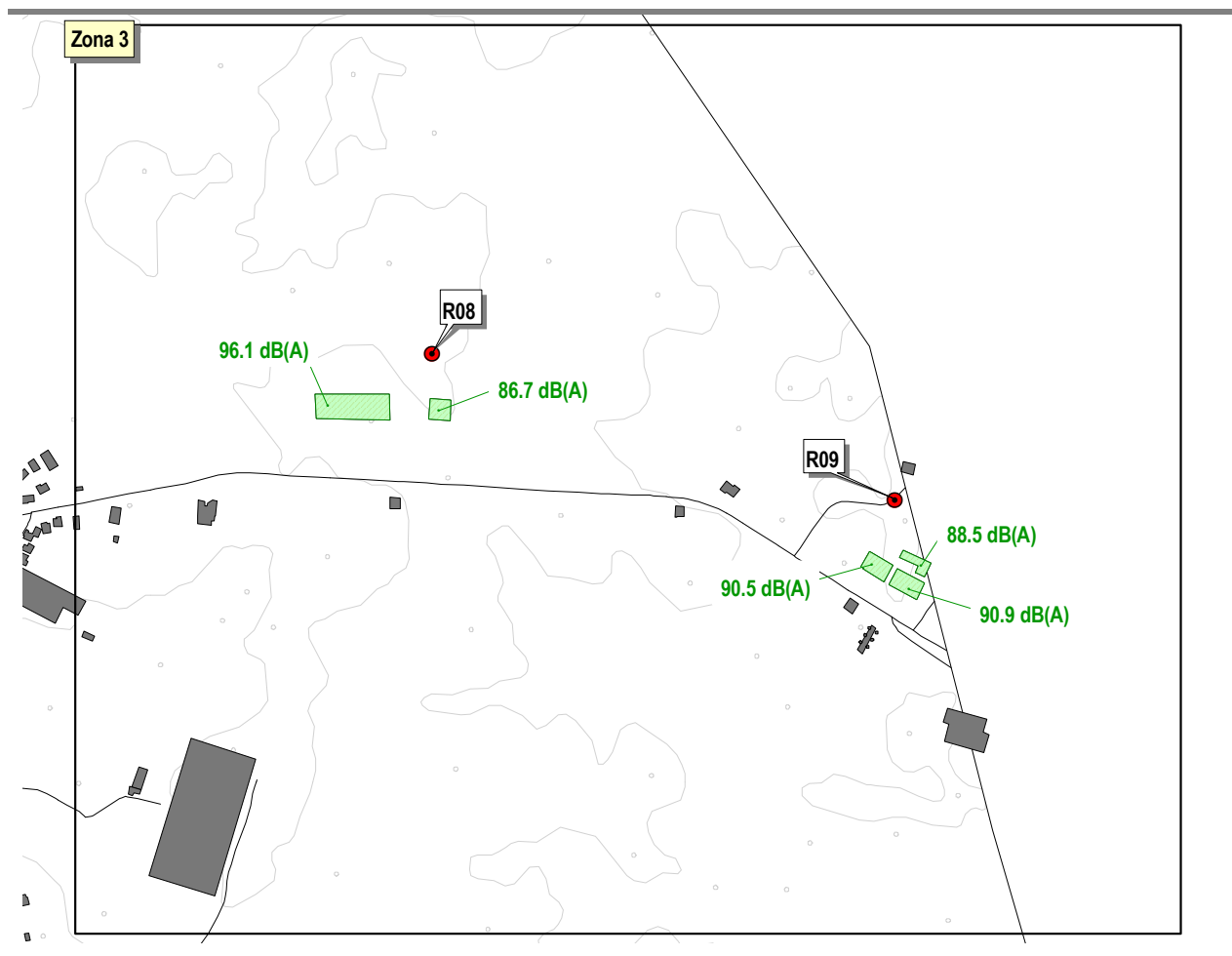
Figura 26 – Esquema representativo da Zona 3 do Concelho da Batalha onde se realizaram medições de Ruído Industrial.
