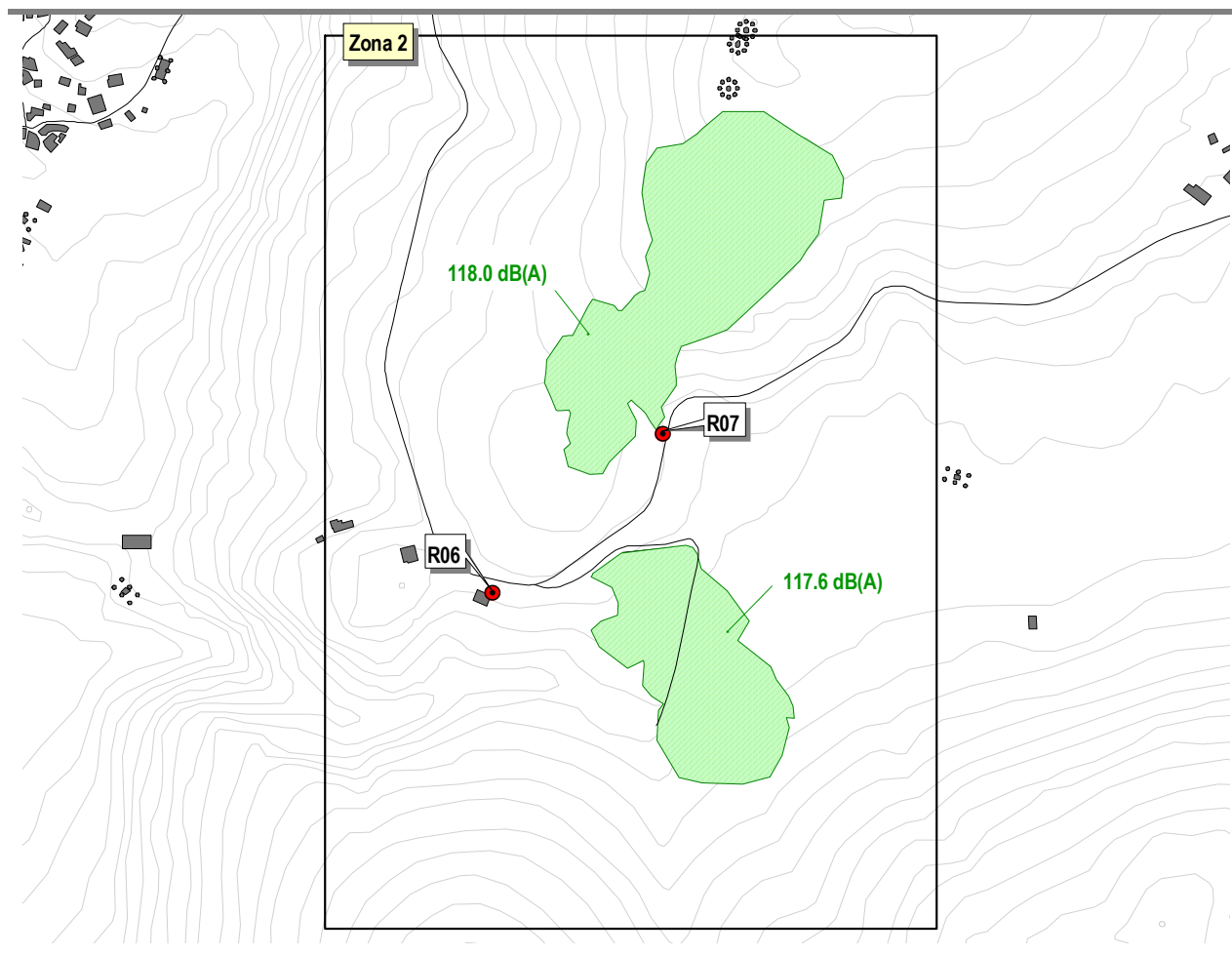
Figura 25 – Esquema representativo da Zona 2 do Concelho da Batalha onde se realizaram medições de Ruído Industrial.
