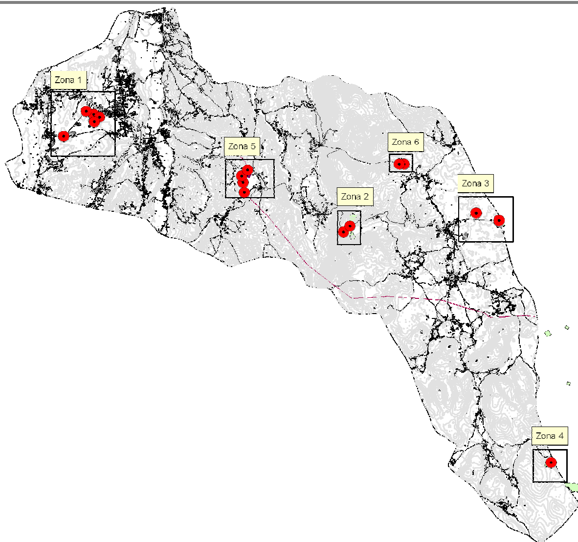
Figura 23 – Localização dos pontos de monitorização de ruído que permitiram aferir a potência das diversas fontes das respectivas unidades/zonas industriais consideradas
