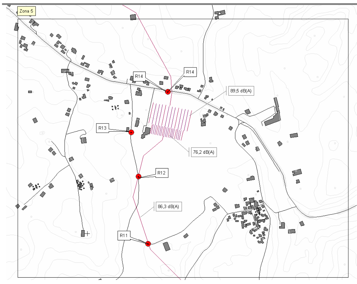
Figura 28 – Esquema representativo da Zona 5 do Concelho da Batalha onde se realizaram medições de Ruído Industrial.
