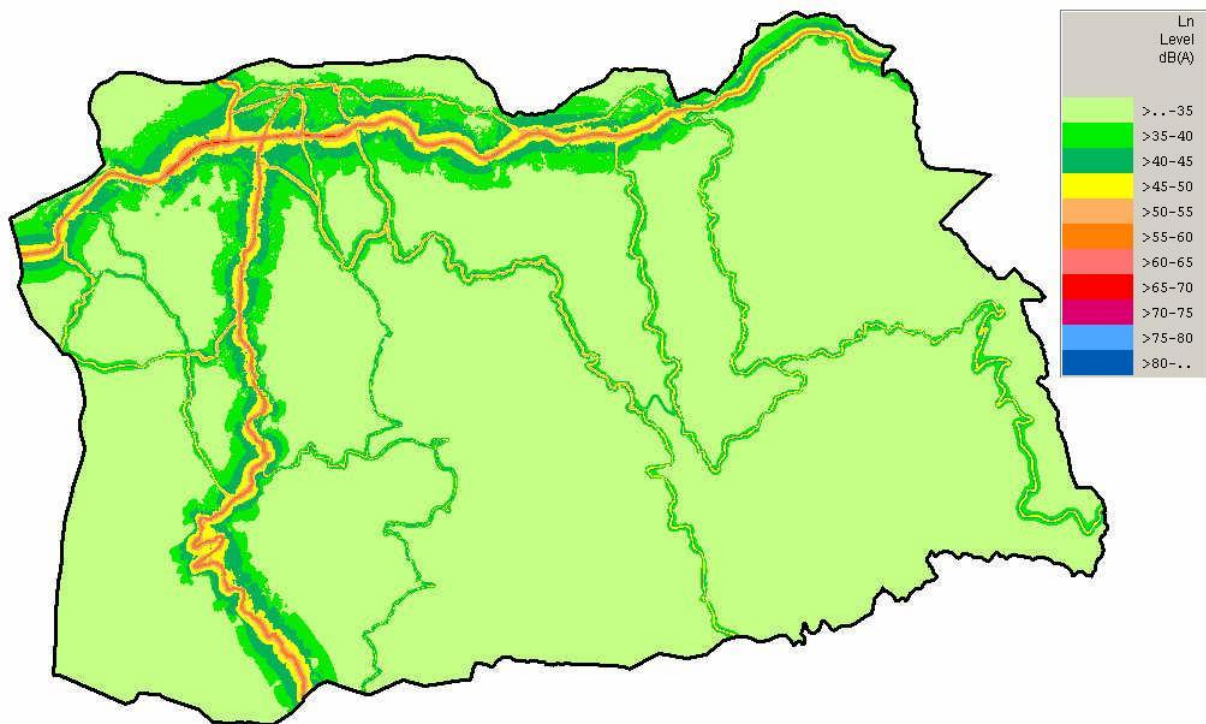
Figura 4: Mapa de Ruído do concelho de Monção - Ano 2008 - indicador de ruído Ln .
