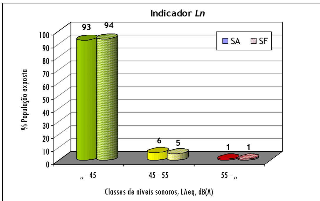
Figura 8: Representação gráfica das estimativas dos níveis de exposição da população do Concelho de Monção ao ruído em termos de Ln (indicador de ruído nocturno).
