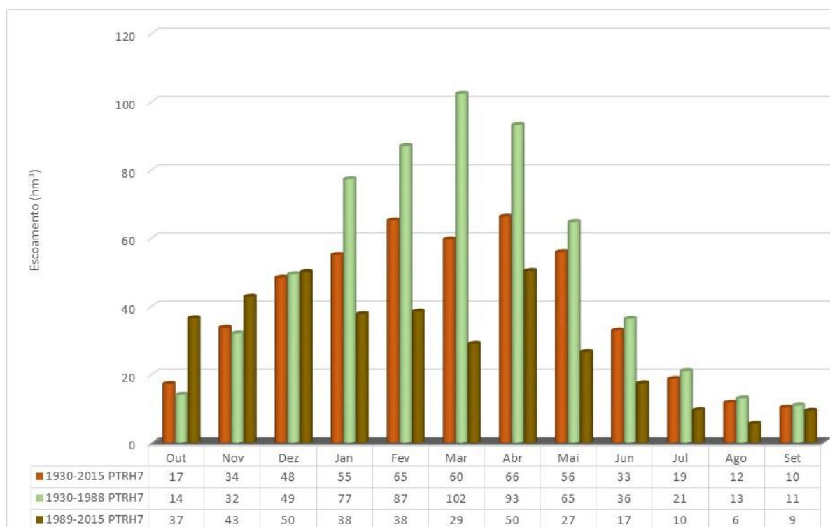
Figura 1.12 – Escocamento médio mensal para o ano seco nos três períodos de análise (1930-2015, 1930-1988 e 1989-2015) na RH
