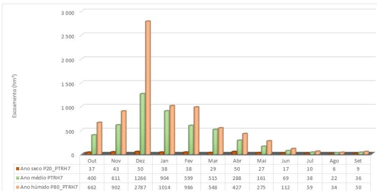
Figura 1.11 – Escocamento médio mensal para os anos húmido, médio e seco para o período de 1989-2015, na RH
