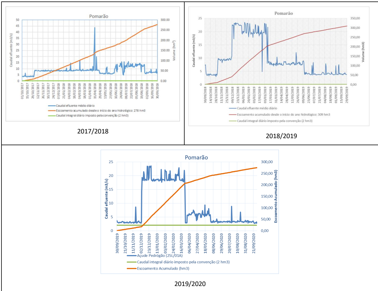
Figura 1.16 – Regime de caudais na estação de controlo de Pomarão.
