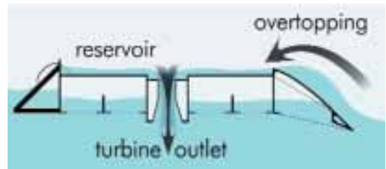
Figura 3.4.14a princípio de funcionamento do Wave Dragon (cortesia Wave Dragon ApS)
