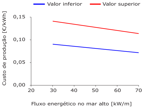
figura 4.3.1 gama de custos de produção de energia eléctrica para centrais costeiras de coluna de água oscilante em função do fluxo médio de energia das ondas no alto mar (Thorpe, 2003).
