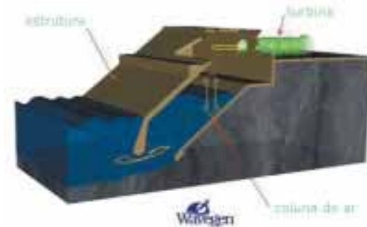
Figura 3.2.1 Esquema de uma central de coluna de água oscilante (cortesia Wavegen)
